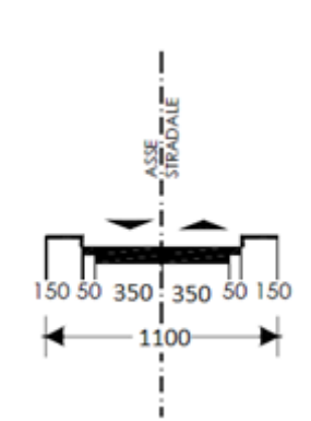
Figura 7 - Sezione tipo di Progetto- Categoria F in ambito urbano con corsie da 3.50m
