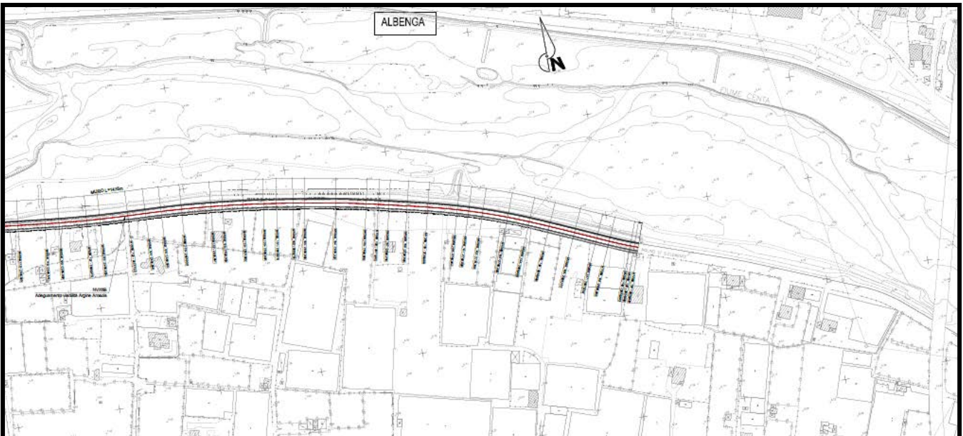
Figura 6 - Stato di Progetto 4/4
