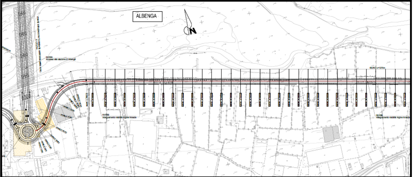
Figura 3 - Stato di Progetto 1/4
