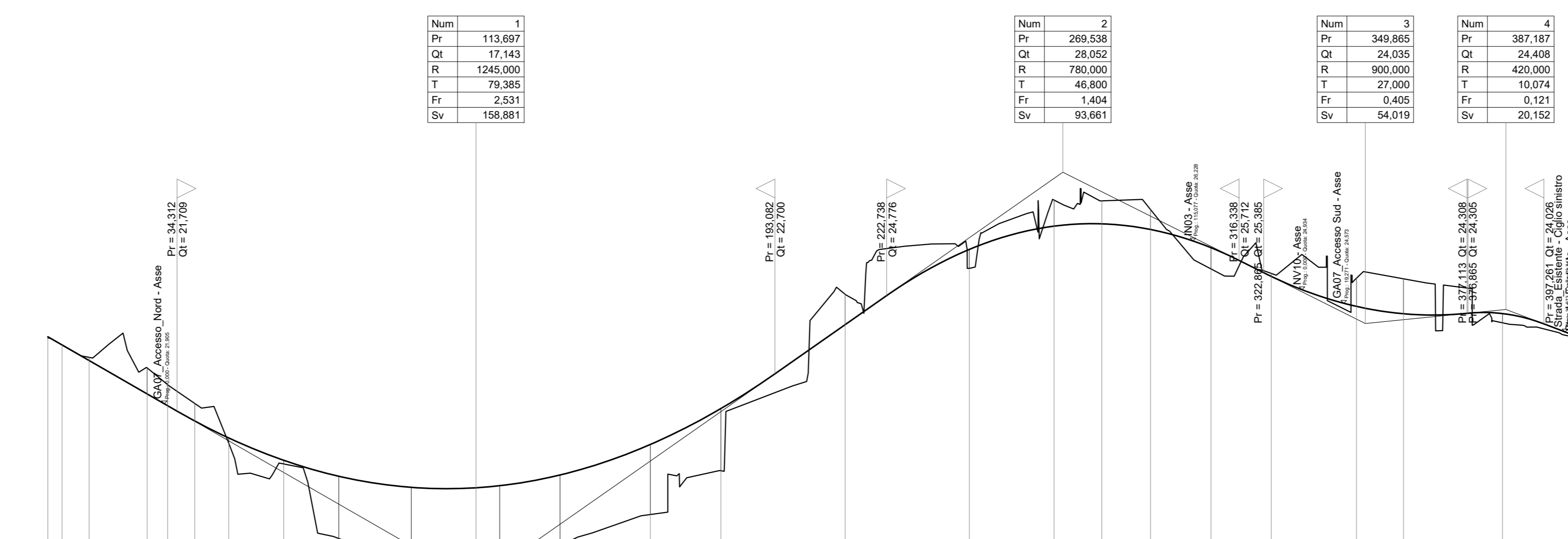
Profilo longitudinale: GA07
