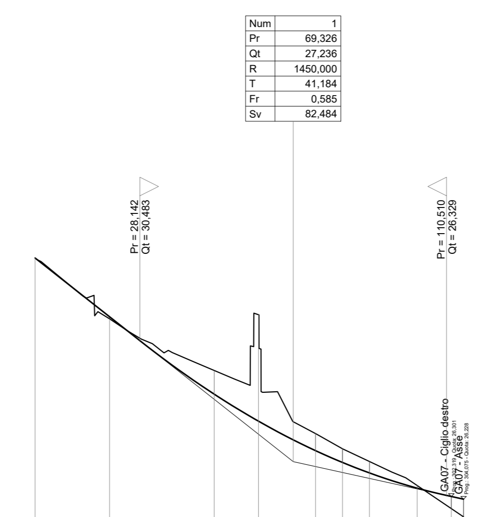
Profilo longitudinale: IN03
