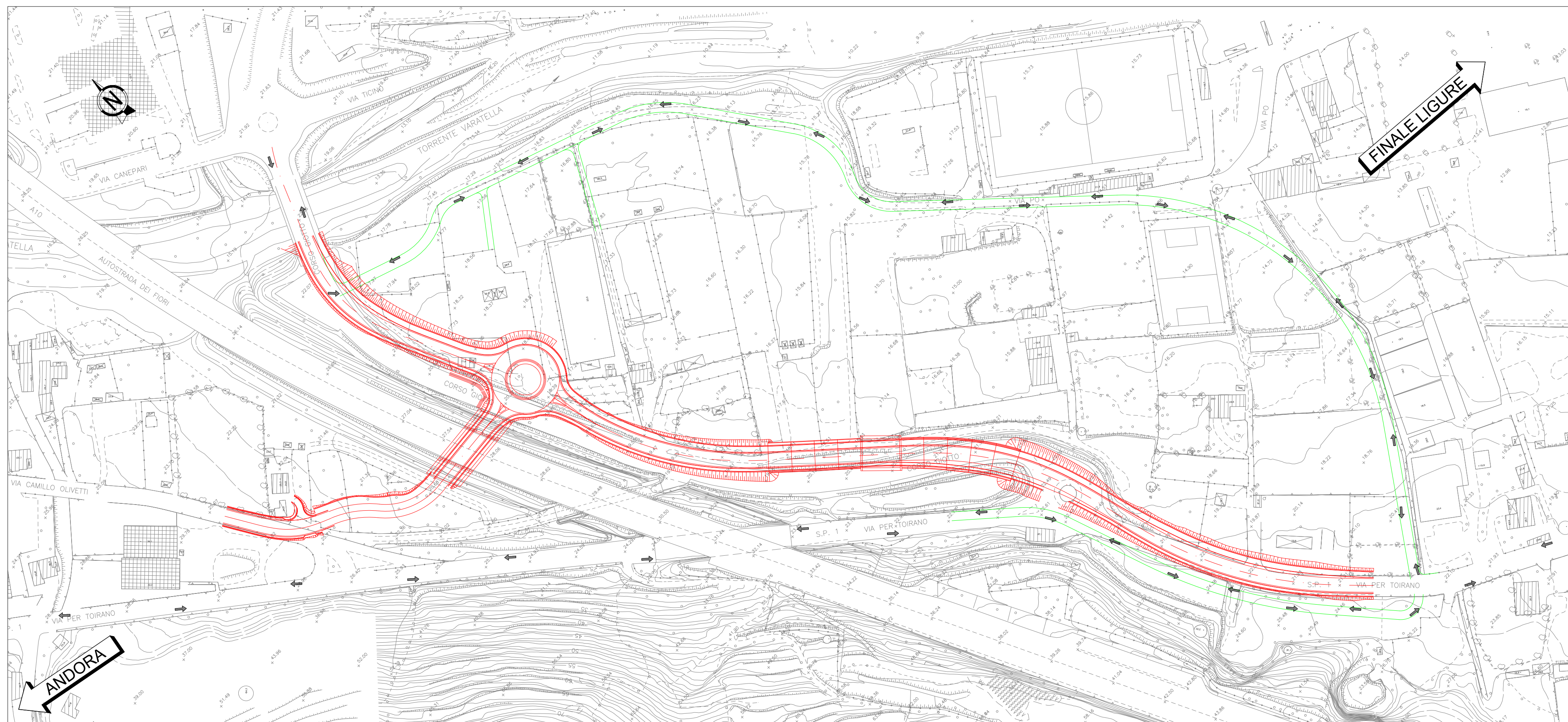
PLANIMETRIA - FASE 2 1:1500
