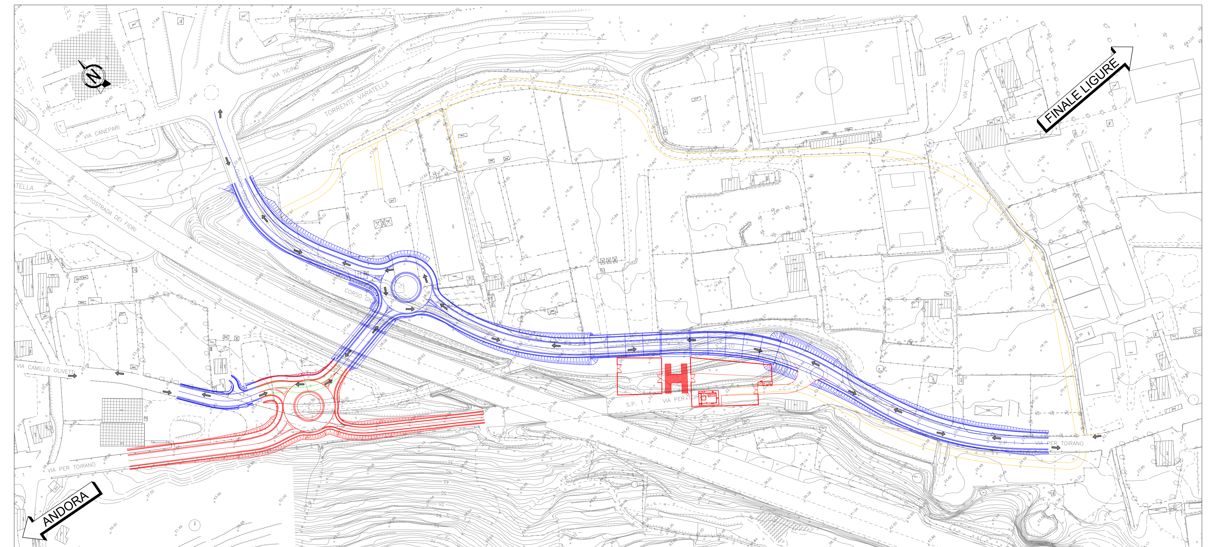
PLANIMETRIA - FASE 3 1:1500
