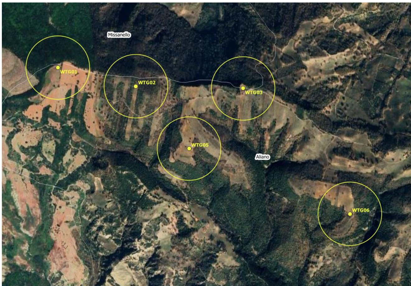
Figura 1 – Indicazione della gittata massima della pala in caso di distacco
