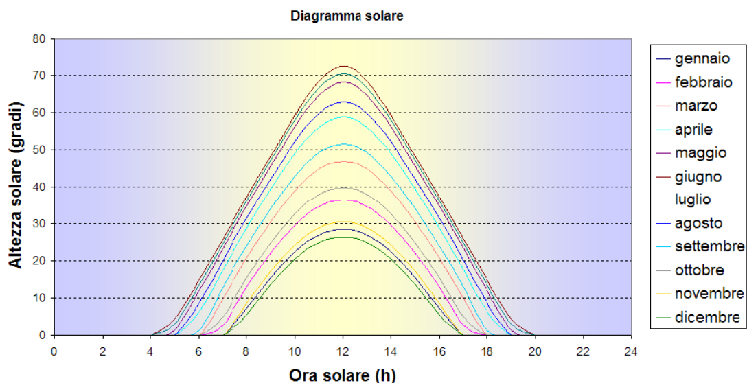
Figura 4-1: Diagramma solare della zona di Aliano
