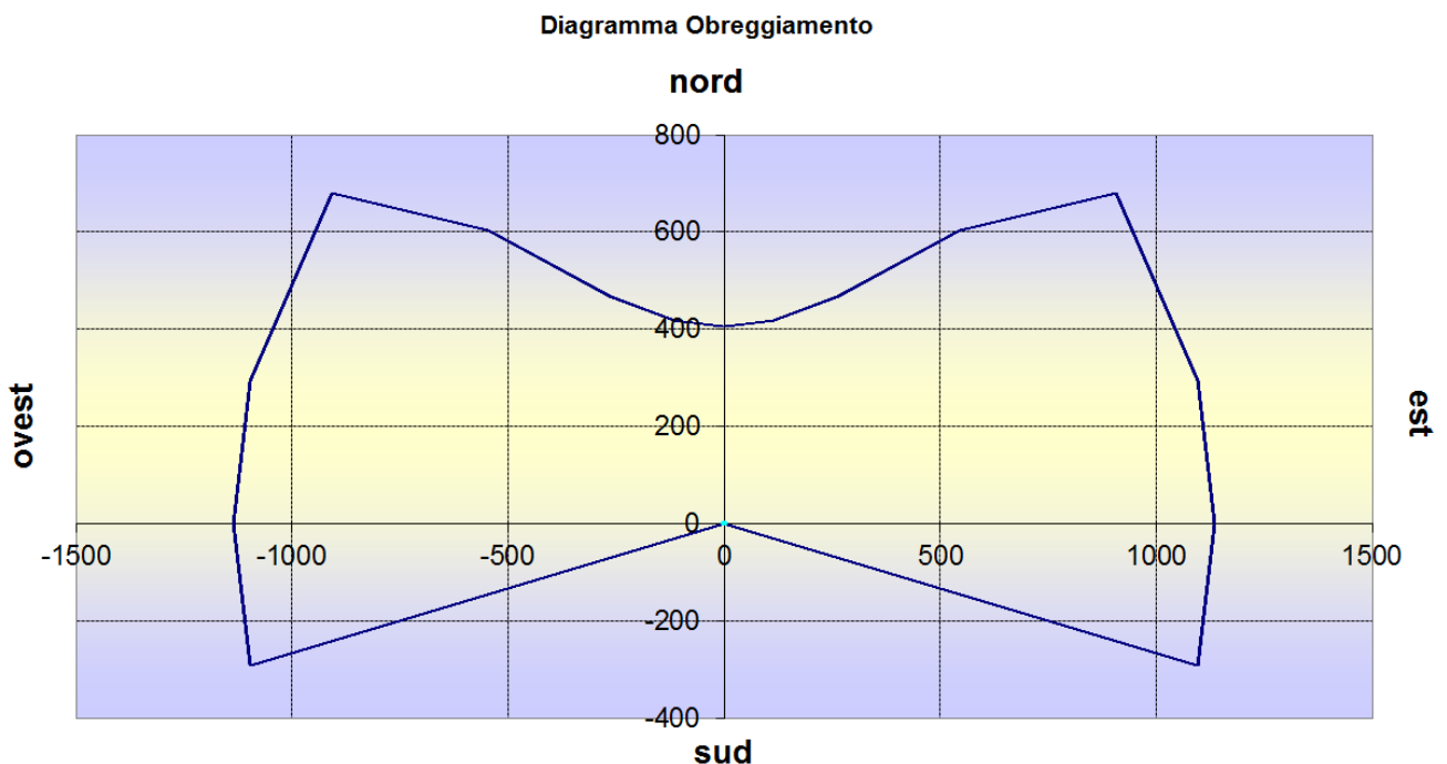
Figura 4-2: Diagramma di ombreggiamento della zona di Aliano (angolo limite 10°)
