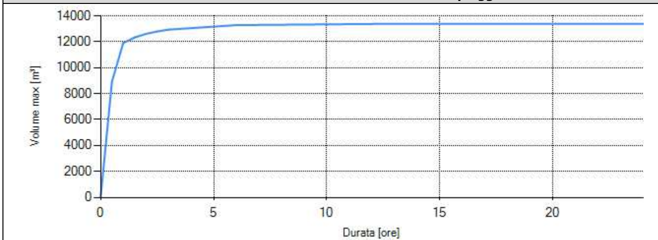
Variatione volume massimo invasato in funzione della durata della pioggia - Grafico
