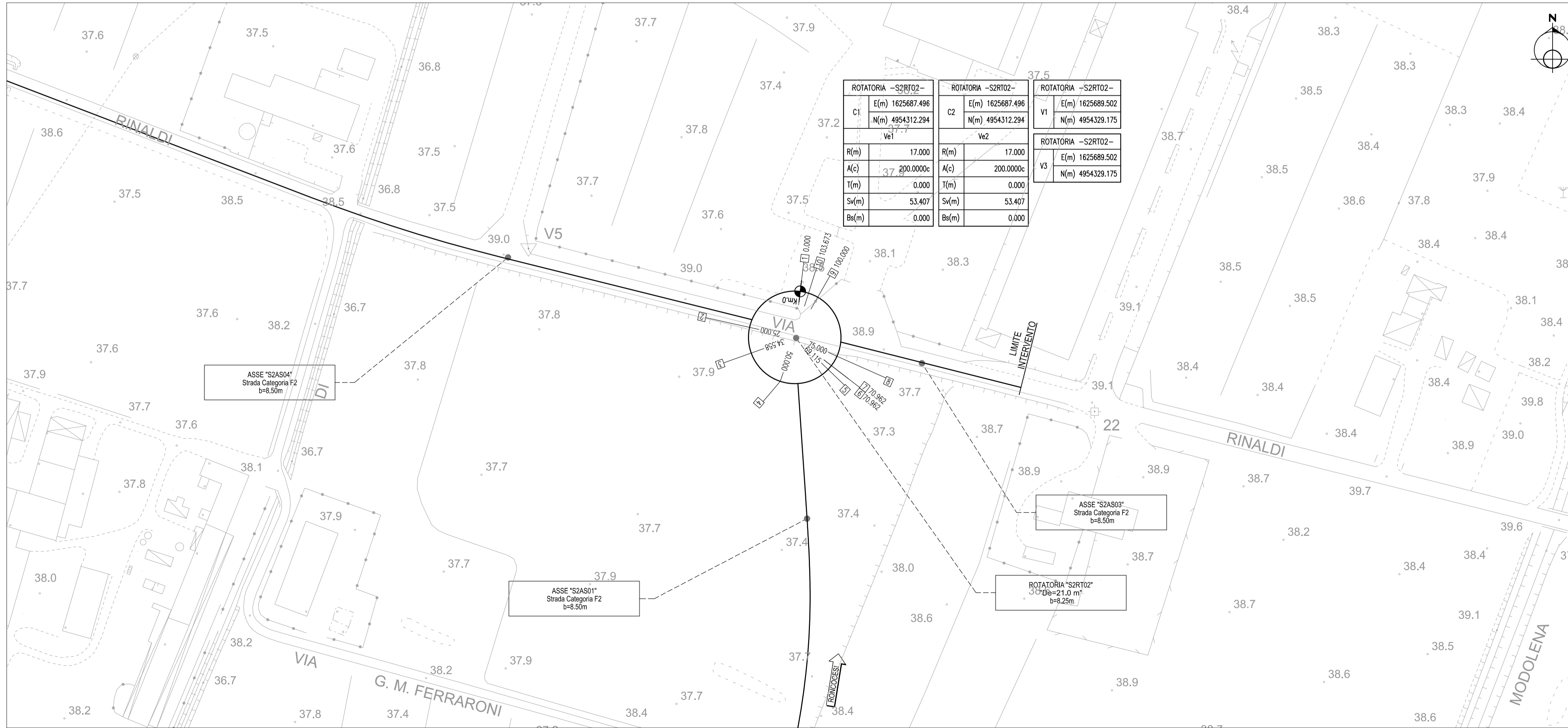
ROTATORIA - S2RT02 - SCALA 1:1000
