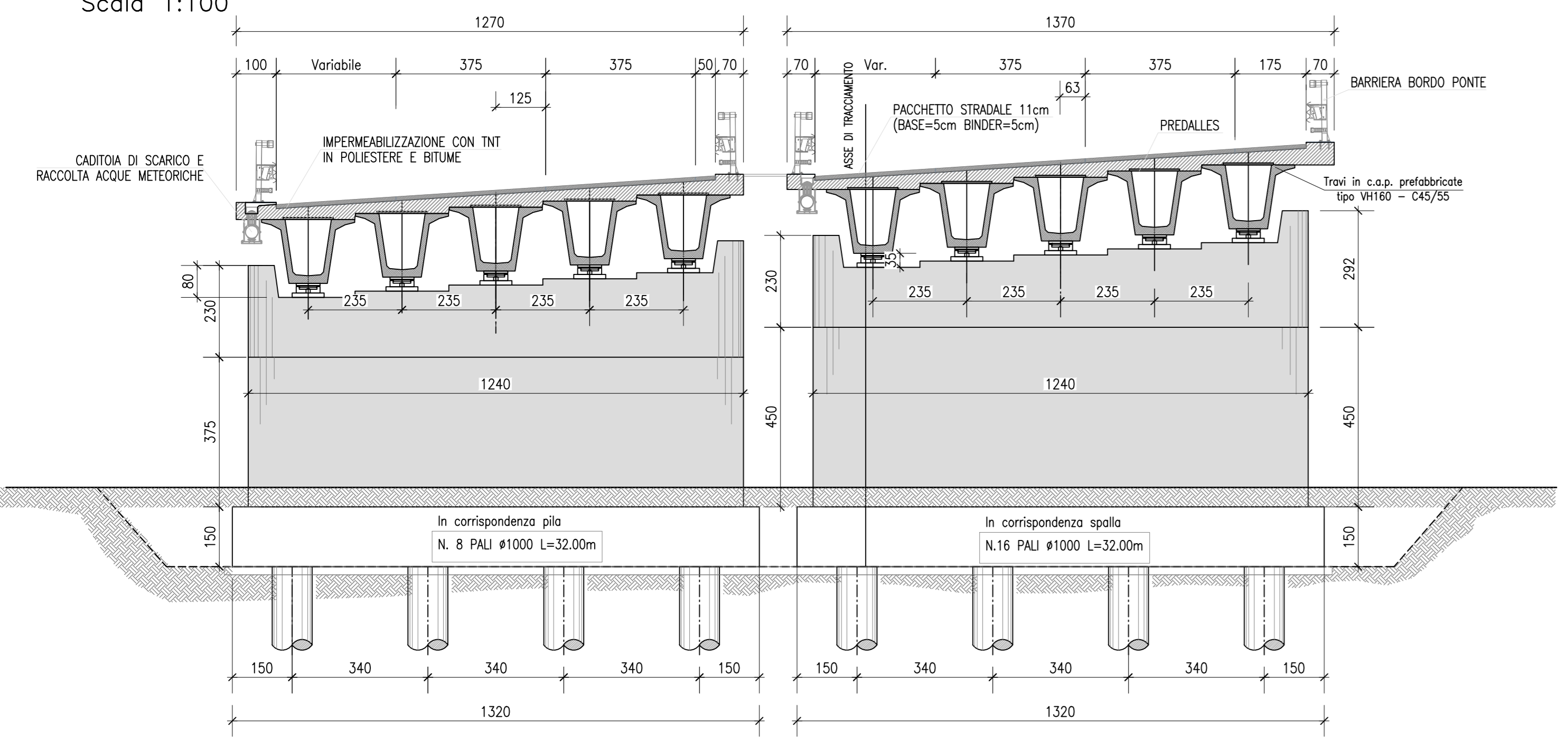
SEZIONE TRASVERSALE IN CAMPATA Scala 1:100
