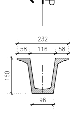
SEZIONE TRAVE IMPALCATO Sez. N-N Scala 1:100
