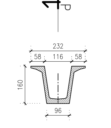
SEZIONE TRAVE IMPALCATO Sez. N-N Scala 1:100
