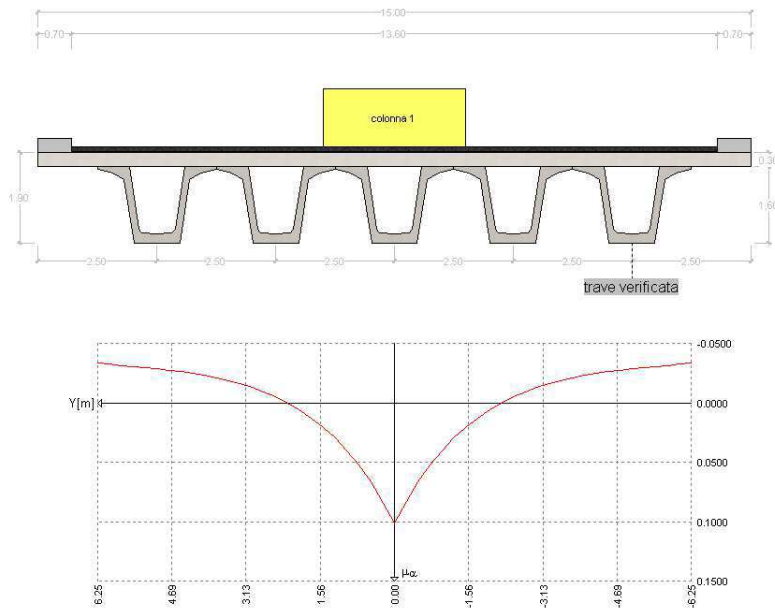
Diagramma coeff. μ di influenza del trasverso, configurazione del carico per M max
