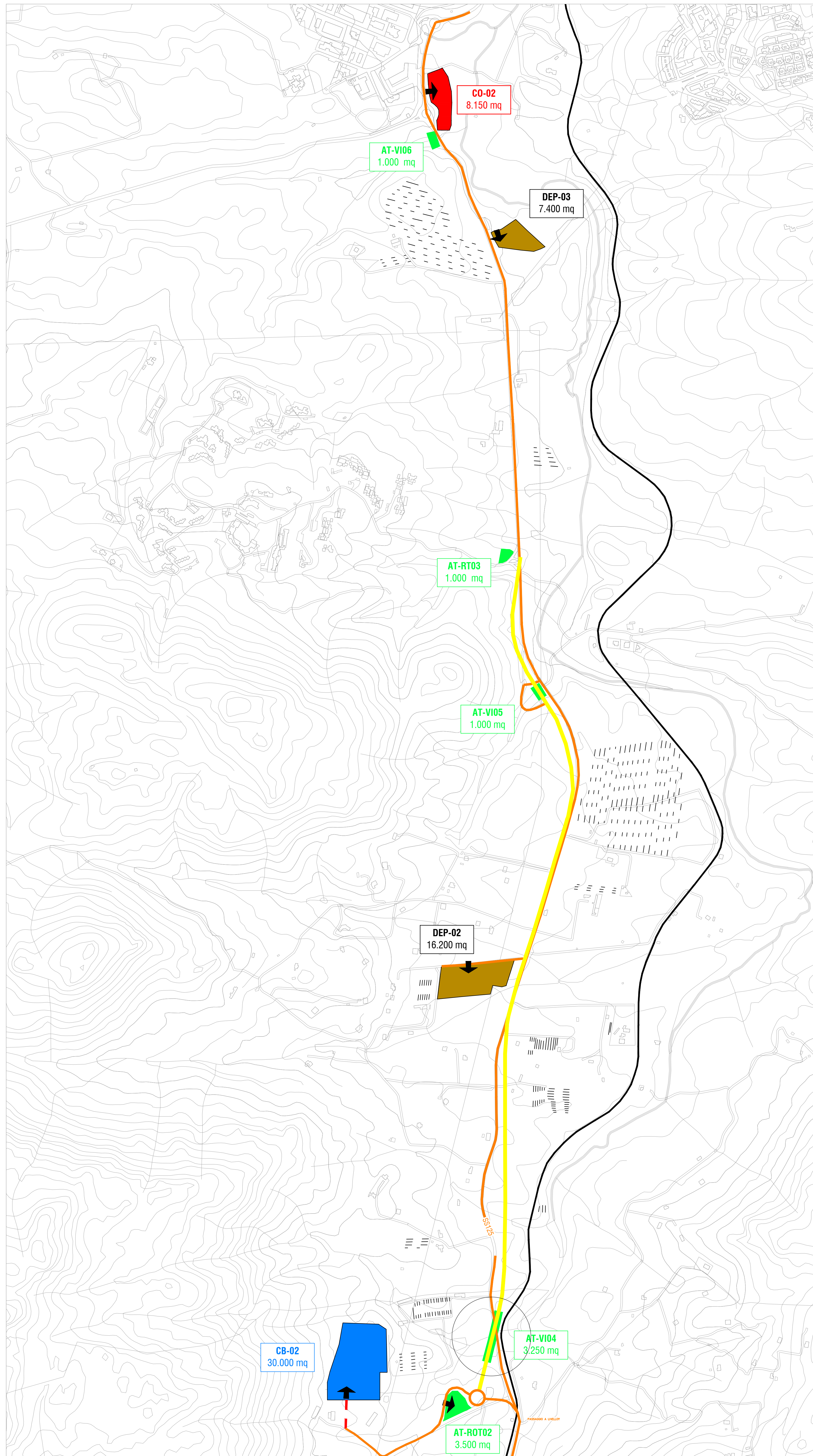
PLANIMETRIA AREE DI CANTIERE E VIABILITA' DI SERVIZIO scala 1:5000
