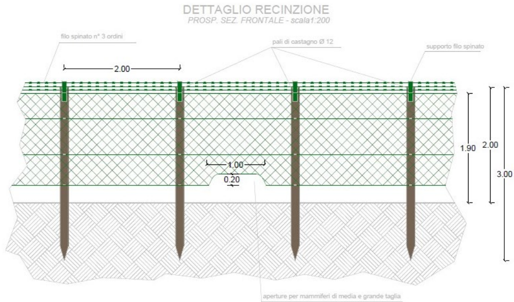
Figura 2: Dettaglio della recinzione di confine area d’impianto
