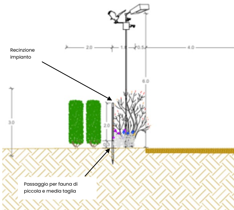
Figura 19 - Particolare palo di videosorveglianza con stalli per uccelli
