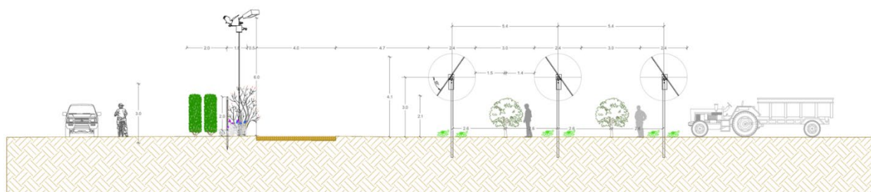
Figura 35 - Particolari strutture tracker
