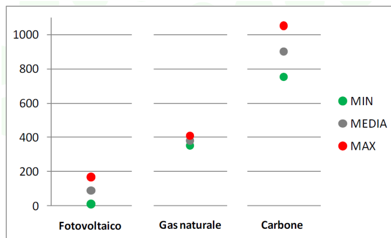
Figura 26 - Valori minimi, medi e massimi per i diversi impianti di produzione dell'energia elettrica
