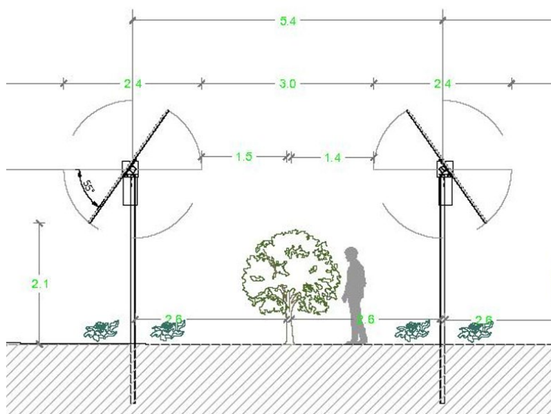
Figura 36 - Sezione strutture tracker
