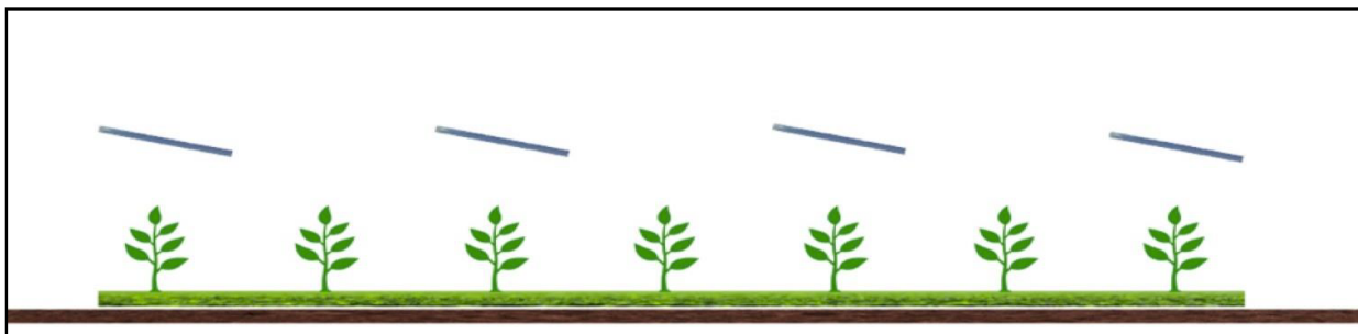
Figura 41 - Configurazione tracker con progetto agricolo al di sotto dei moduli (Fonte: Linee guida in materia di impianti agrovoltaici)
