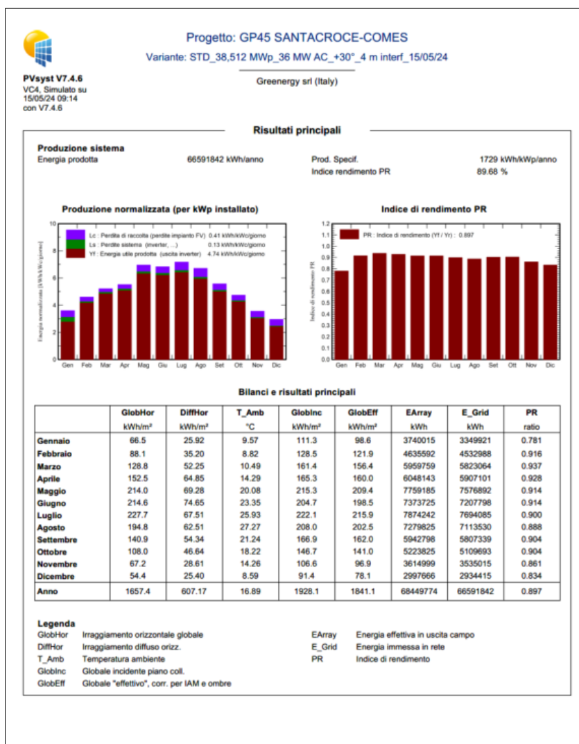
Figura 39 - Analisi della producibilità tramite PVSyst relativa alla tipologia di impianto standard
