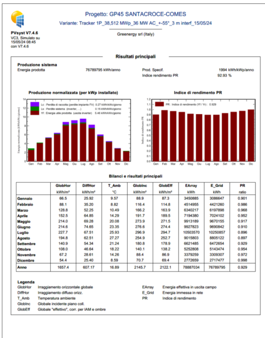
Figura 40 - Analisi della producibilità tramite PVSyst relativa alla tipologia di impianto agrivoltaico
