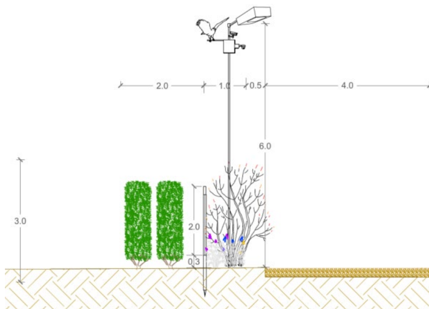
Figura 30 - Particolare palo di videosorveglianza con stallo per uccelli
