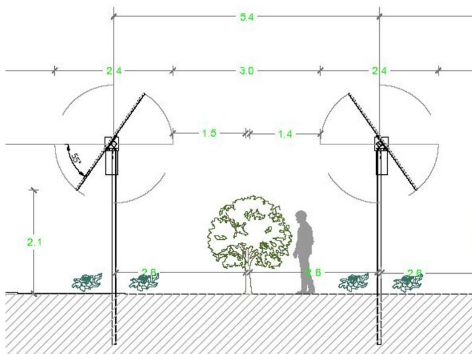
Figura 42 - Particolare sezione struttura tracker inclinata a 55^\circ - impianto standard
