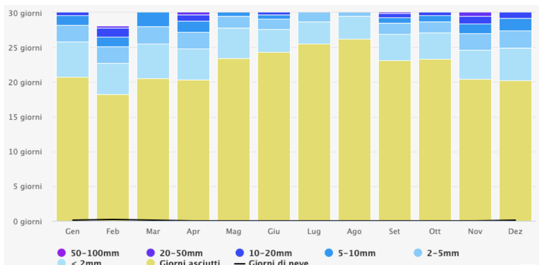
Figura 23 - Andamento annuo delle precipitazioni
