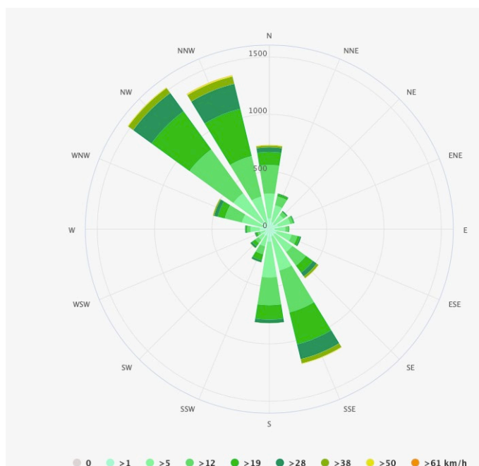
Figura 25 - Diagramma esplicativo intensità del vento
