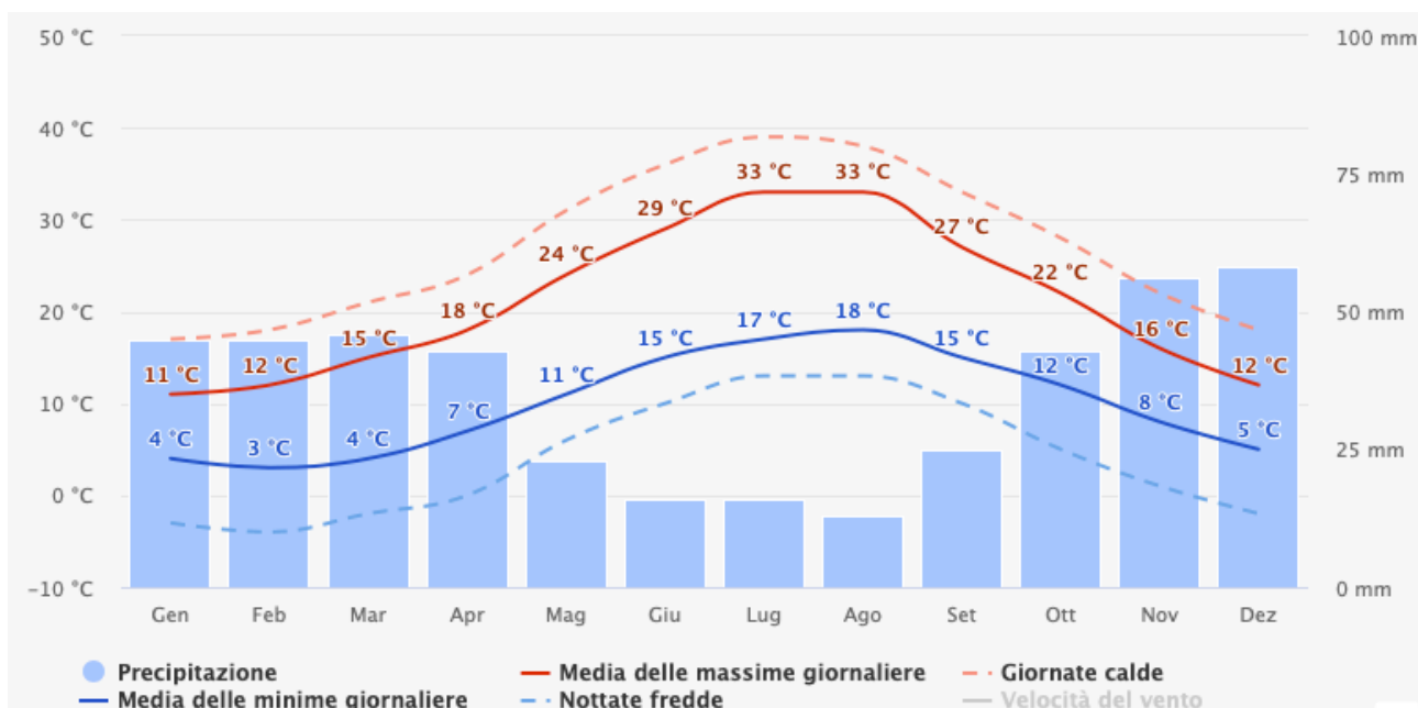
Figura 21 - Andamento delle temperature annuali nel Comune di Castellaneta
