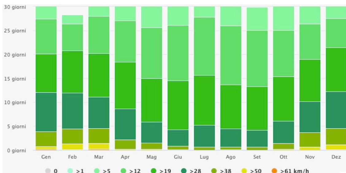
Figura 24 - Diagramma della velocità del vento mensile nel Comune di Castellaneta
