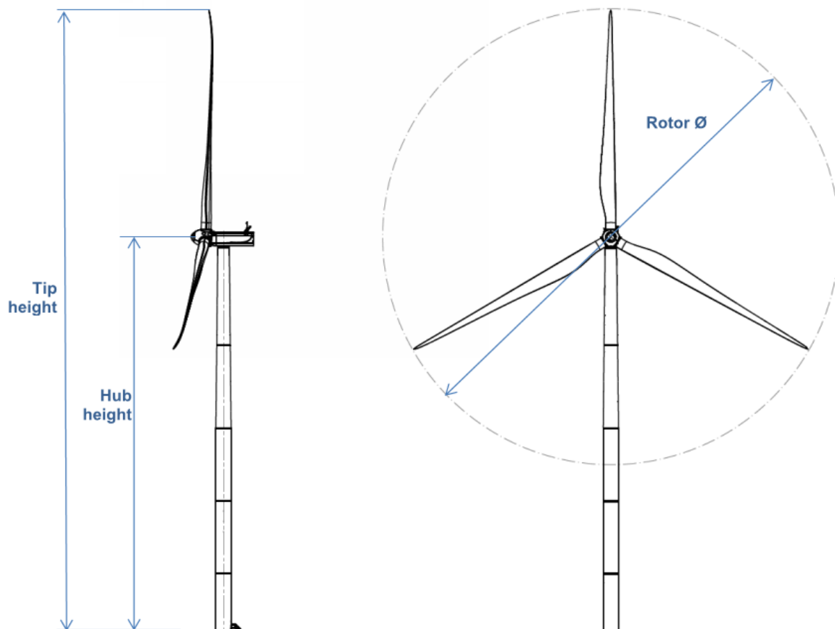
Figura 6.2 – Aerogeneratore tipo Siemens - Gamesa SG 6,2-170 AM0 altezza al mozzo 135 m, e diametro rotore di 170 m
