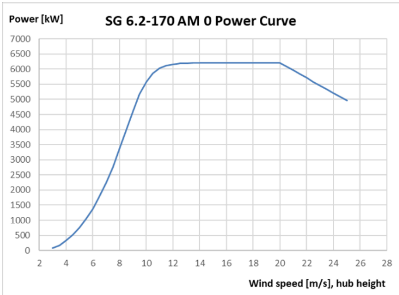
Figura 6.3 – Dati di potenza generatore tipo SG 6.2-170 AM0
