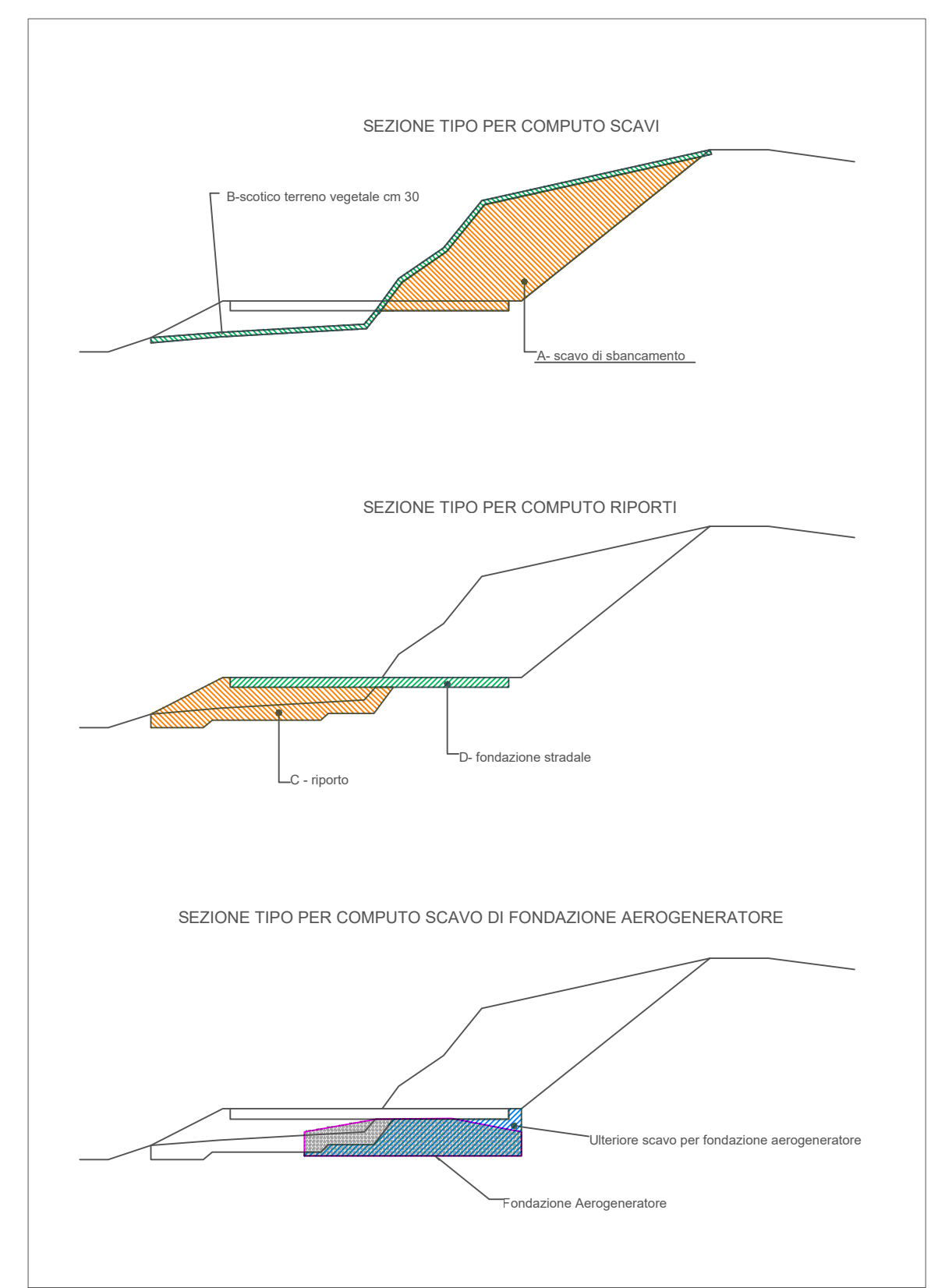
SCHEMA PER IL CALCOLO DEI VOLUMI
