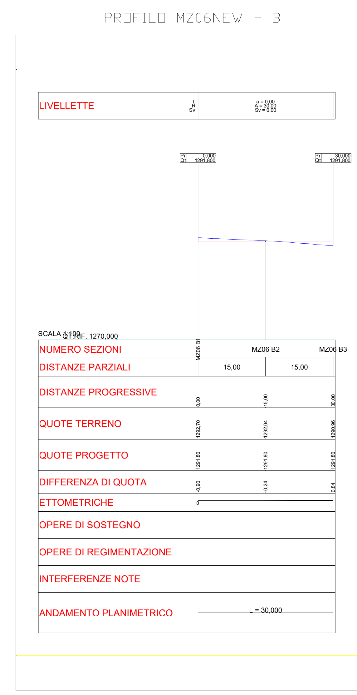
PROFILI LONGITUDINALI PIAZZOLA Scala 1:500
