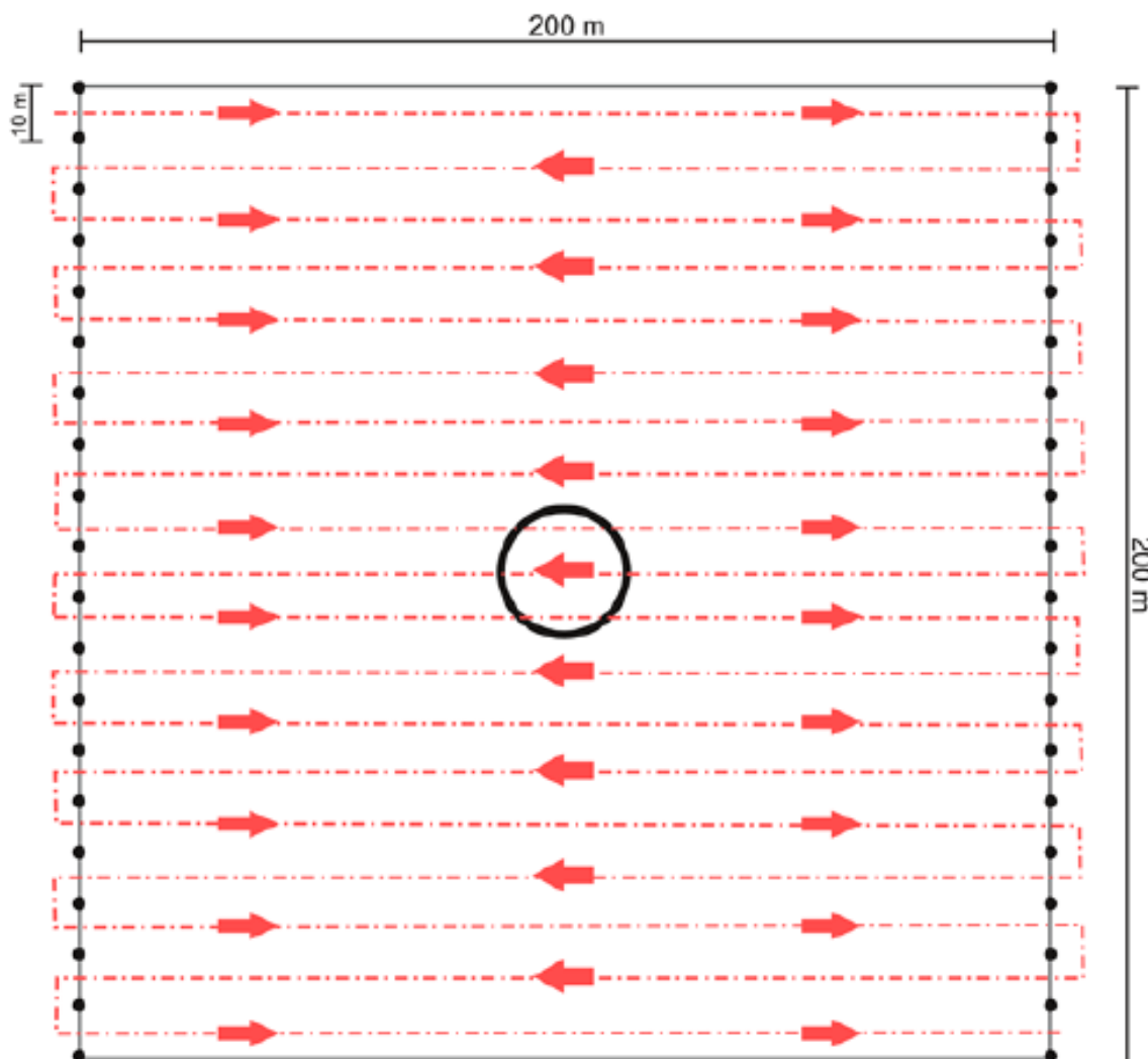
Figura 12: Schema del transetto (in rosso) da eseguire per la ricerca carcasse intorno alla torre eolica (cerchio nero)
