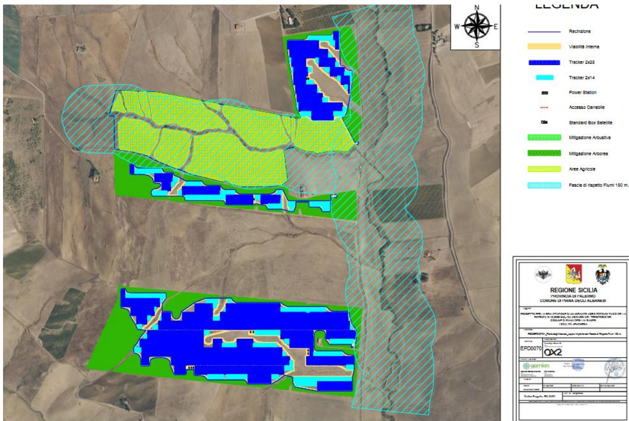
Figura 4 - "Layout impianto con fascia di rispetto Fiume 150" (RS06EPD007011).
