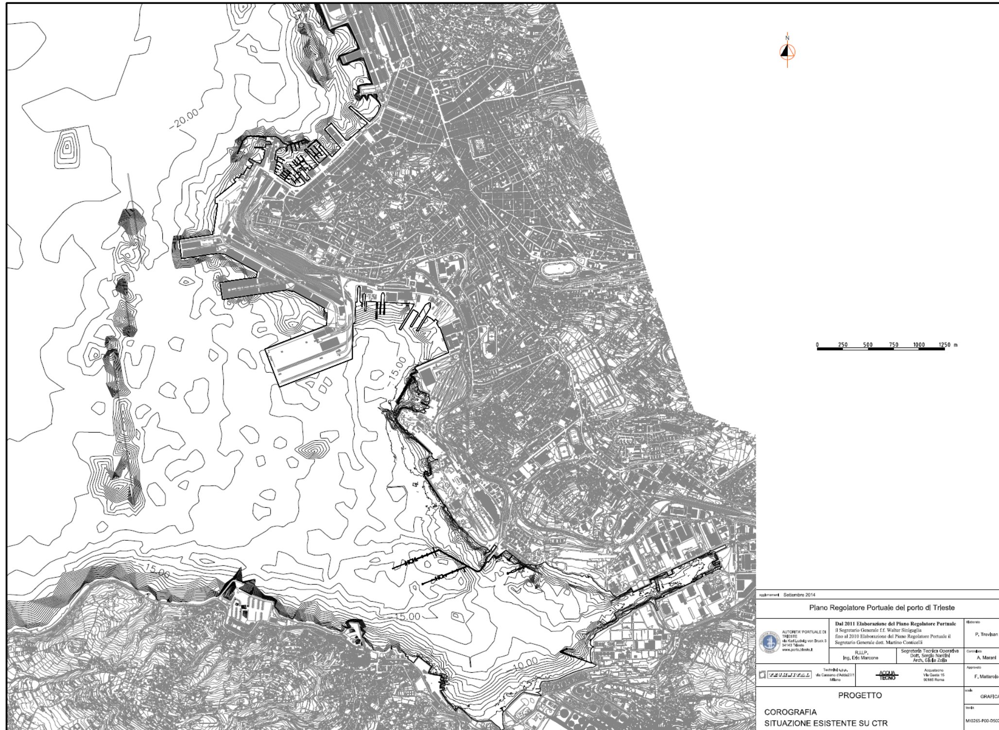
FIGURA 2-2 – PLANIMETRIA GENERALE DEL PORTO DI TRIESTE.
