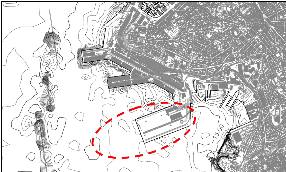
FIGURA 3-2 – LOCALIZZAZIONE DEL COMPLETAMENTO PROLUNGAMENTO DEL MOLO VII
