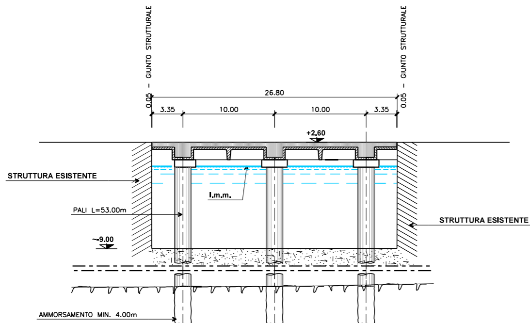
SEZIONE D-D - OPERA-13 ARSENALE SAN MARCO
