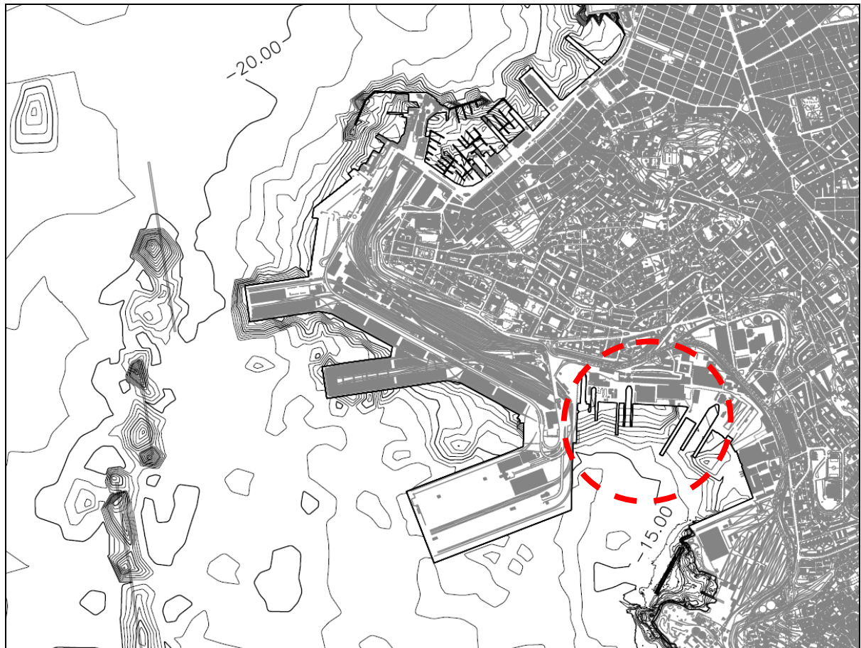
FIGURA 3-2 – LOCALIZZAZIONE DELL'AMPLIAMENTO BANCHINE ARSENALE SAN MARCO
