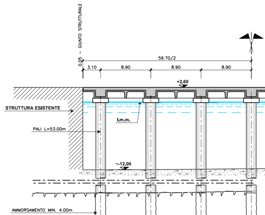
SEZIONE E-E - OPERA-13 ARSENALE SAN MARCO
