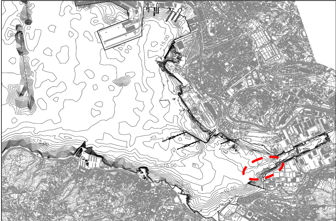
FIGURA 3-2 – LOCALIZZAZIONE DEL COMPLETAMENTO DEL BANCHINAMENTO DEL TERMINAL RO-RO NOGHERE, CON REALIZZAZIONE DELLA CASSA DI COLMATA E
