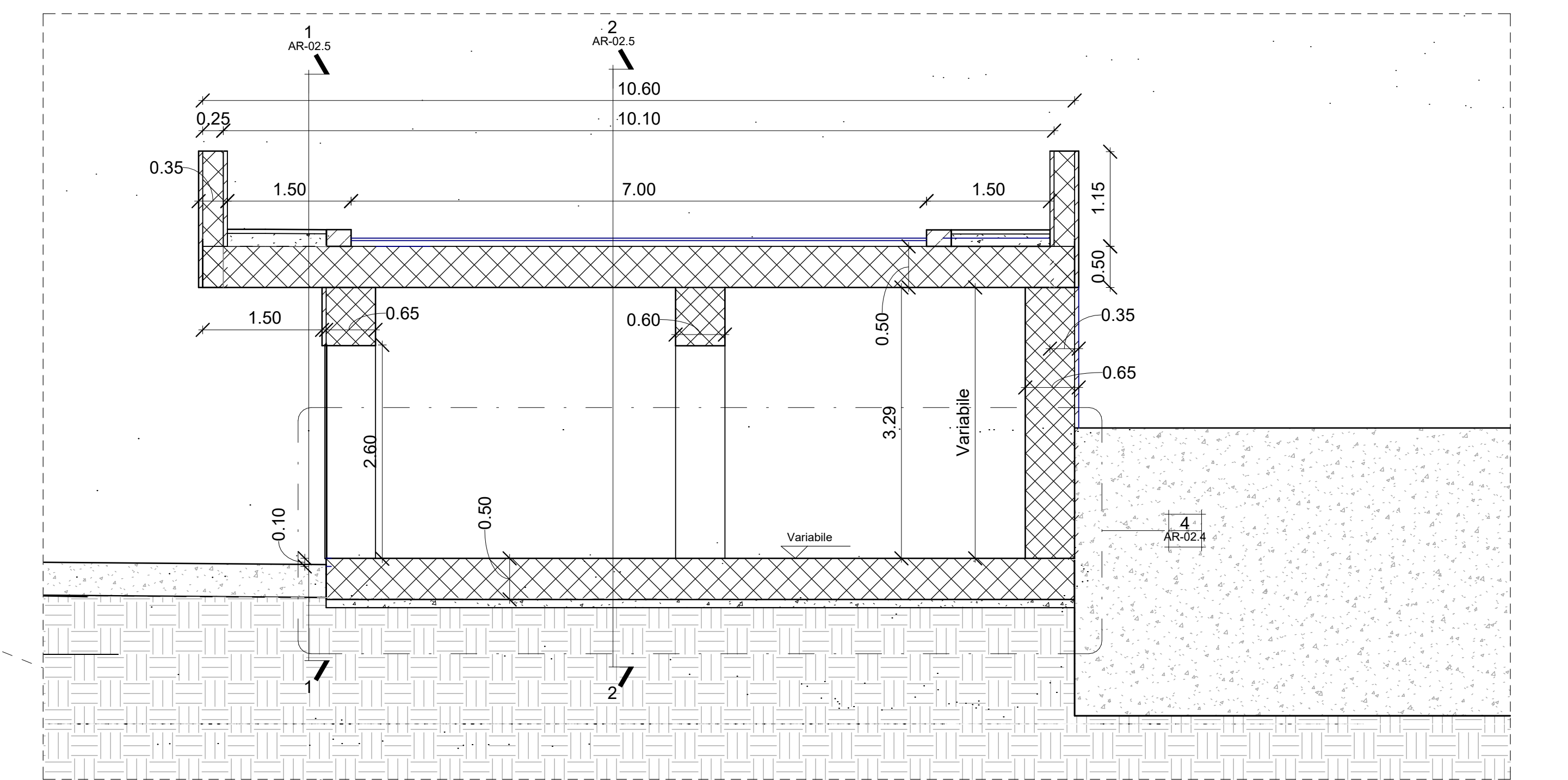
SEZIONE TRASVERSALE RAMPA 3-3
