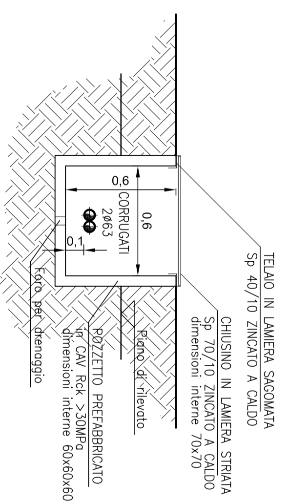
PARTICOLARE POZZETTO DI ISPEZIONE SU CAMDOTTO ILLUMINAZIONE
