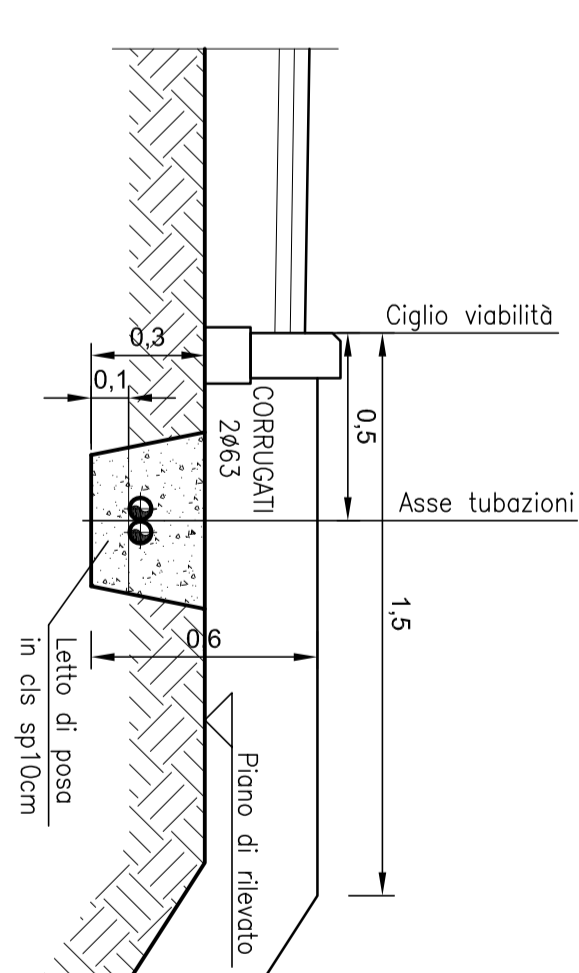
PARTICOLARE CAVIDOTTO ILLUMINAZIONE
