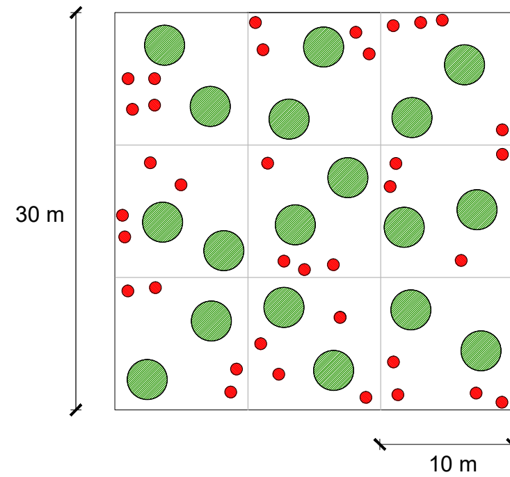
Schema d'impianto (nelle zone aperte in assenza di Pini domestici e arbusti compatibili con la pineta)
