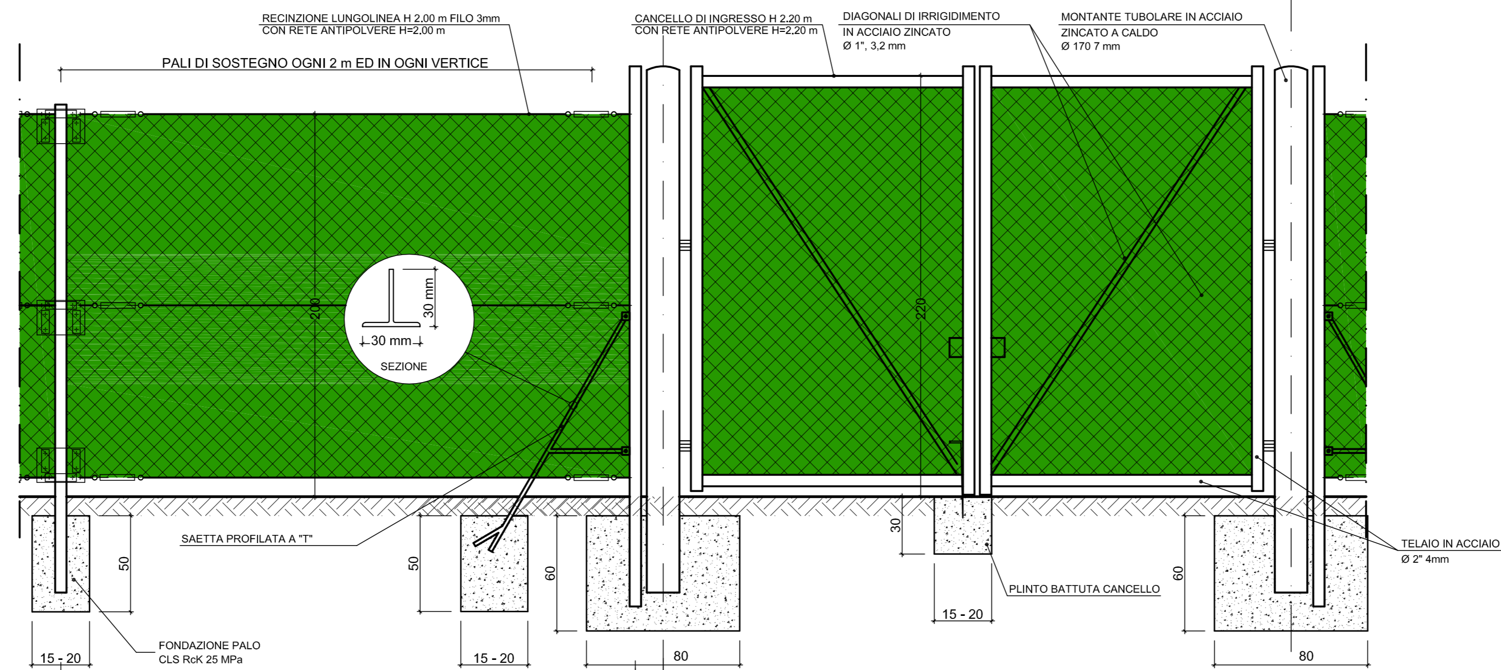
CANCELLO PASSO CARRABILE SCALA 1:20 VISTA FRONTALE
