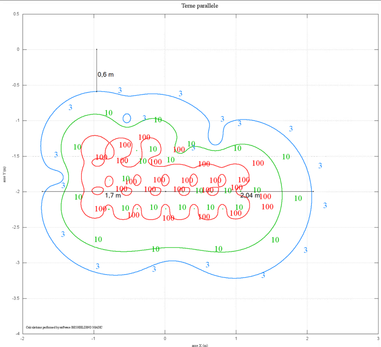
Figura 5 – Curve di iso-campo dell'induzione magnetica B
