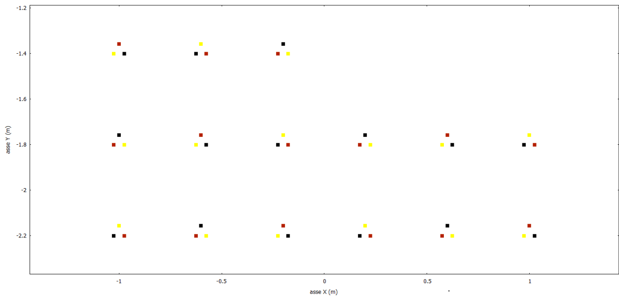
Figura 4 – Disposizione cavi AT nello spazio – Simulazione mediante software BE Shielding MAGIC - Magnetic Induction Calculation,
