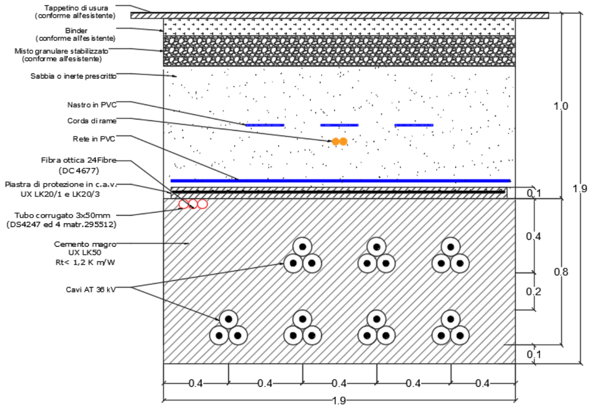
Figura 1 - Tipico di sezione cavidotto AT composto da sette terne di cavi su strada asfaltata
