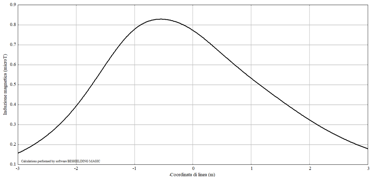
Figura 6 – Valori dell'induzione magnetica B sul livello stradale.
