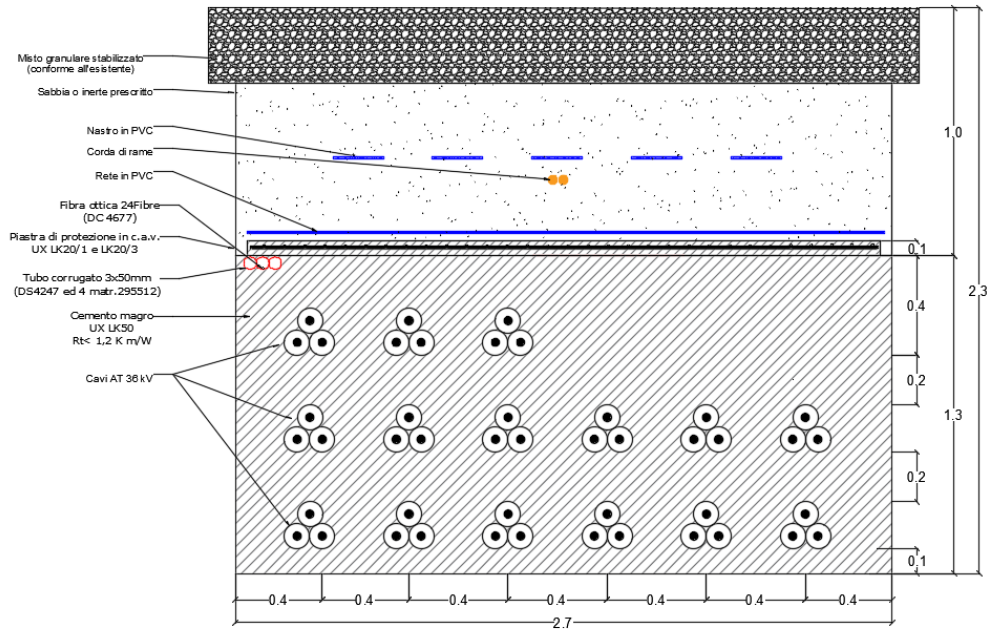
Sezione B15-B15' - Quindici terne di cavi 36 kV su strada bianca Scala 1:100
