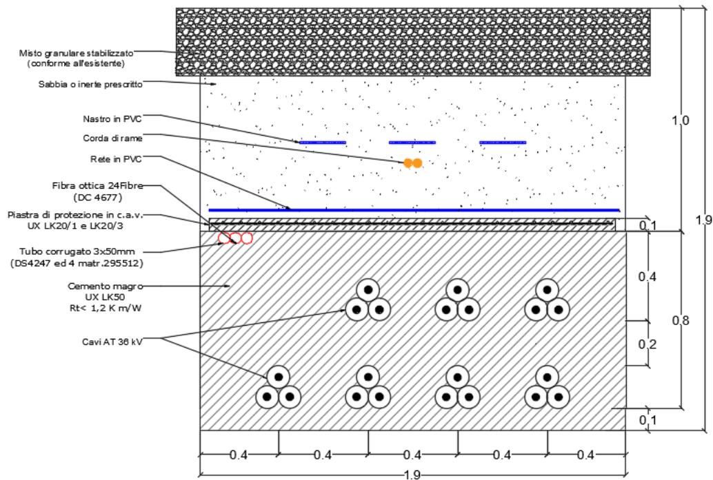
Figura 2 - Tipico di sezione cavidotto AT formato da sette teme di cavi su strada sterrata
