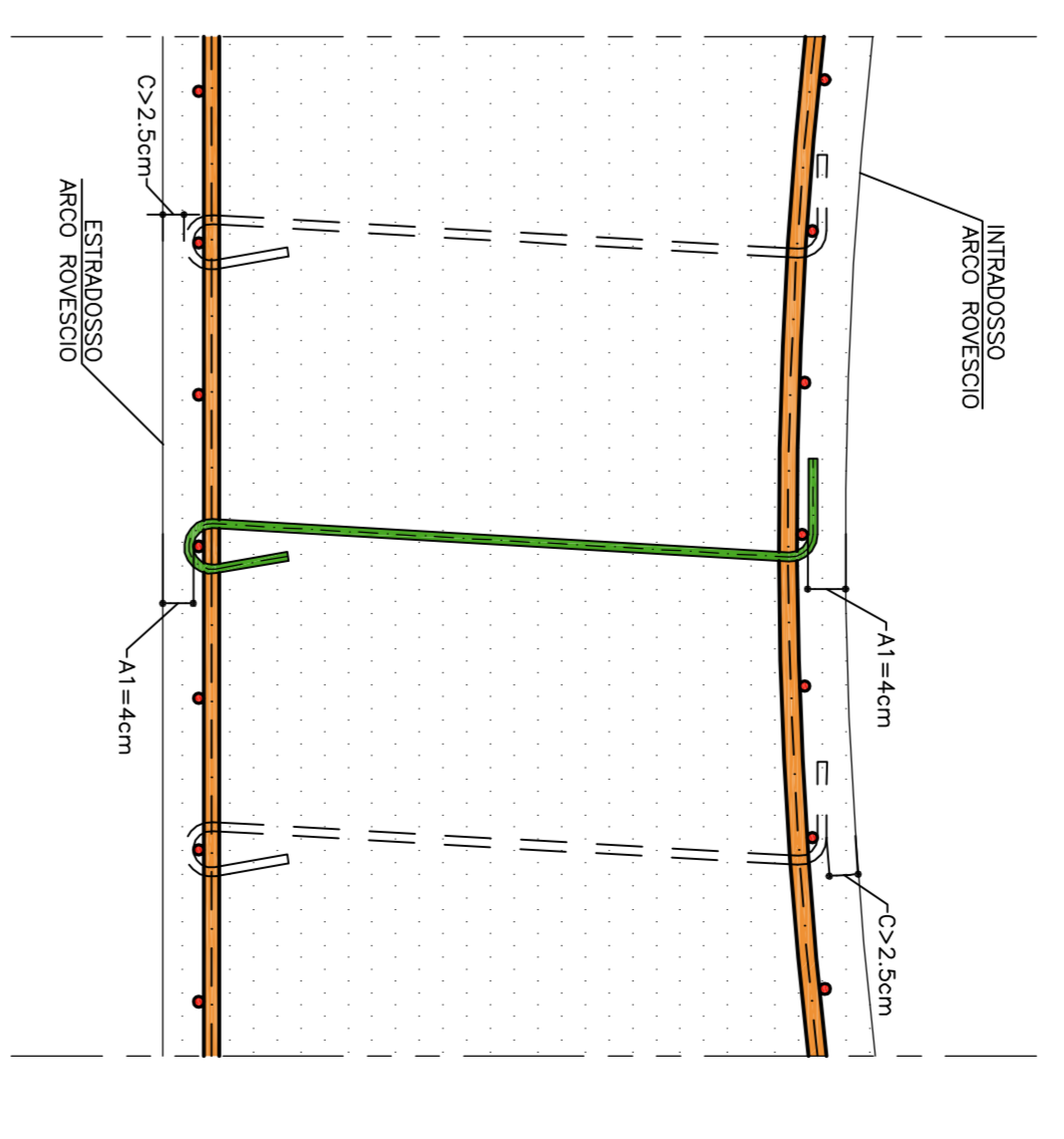
PARTICOLARE COPRIFERRO ARCO ROVERSCIO
