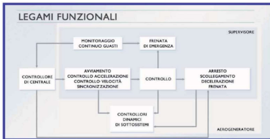
Figura 1.1: Schema di controllo e supervisione dell'aerogeneratore
