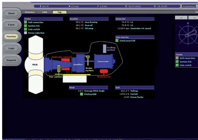
Figura 1.3: Monitoraggio remoto di una turbina eolica in funzione
