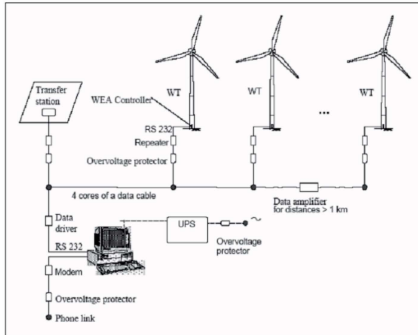
Figura 1.2: Schema logico del funzionamento del sistema SCADA
