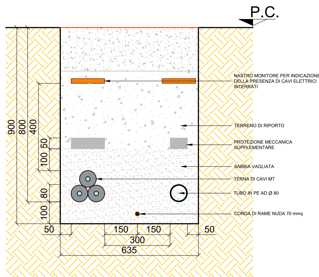
TIPICO SEZIONE DI SCAVO "TIPO A" POSA DI SINGOLA TERNA DI CAVI MT, LINEE DI SEGNALE E CORDA DI RAME NUDA INTERRATI SCALA 1:10
