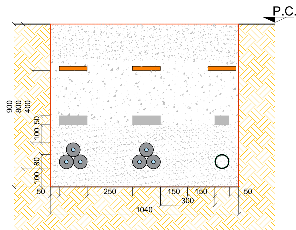
TIPICO SEZIONE DI SCAVO "TIPO B" POSA DI n.2 TERNE DI CAVI MT, LINEE DI SEGNALE E CORDA DI RAME NUDA INTERRATI SCALA 1:10
