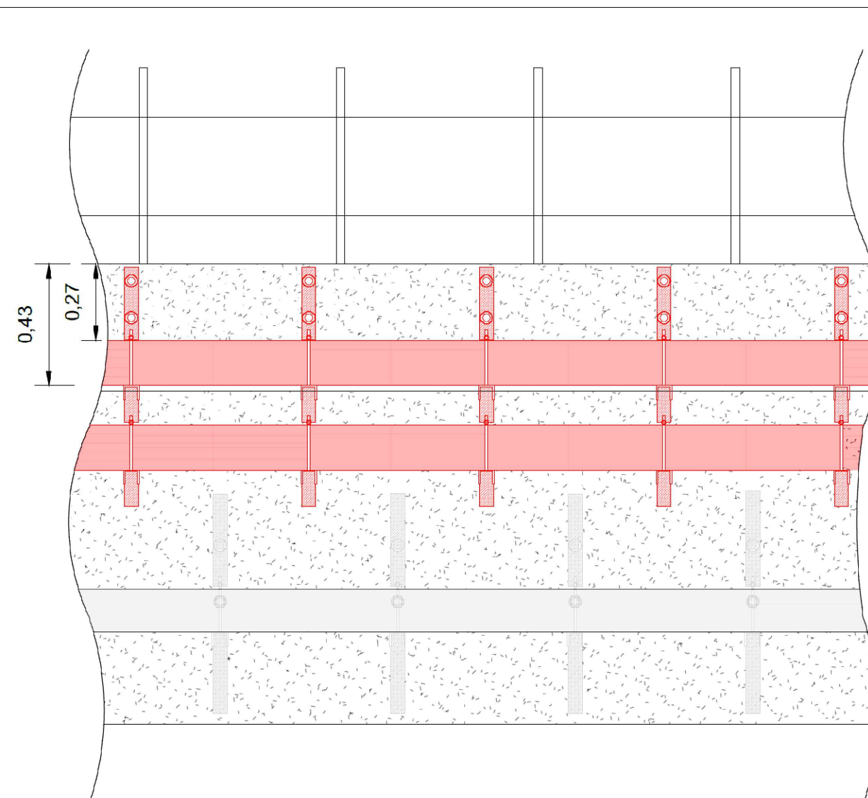
VISTA LONGITUDINALE
