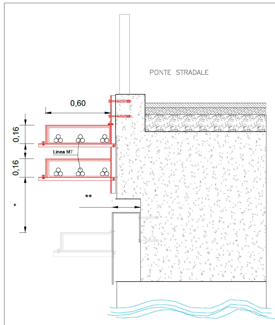
VISTA IN SEZIONE
