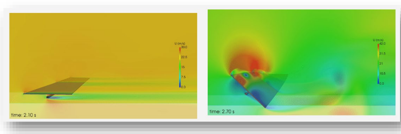
Figura 4 Simulazioni CFD eseguite da Soltec in collaborazione con Lynx basate sulla metodologia Dy-Wind
