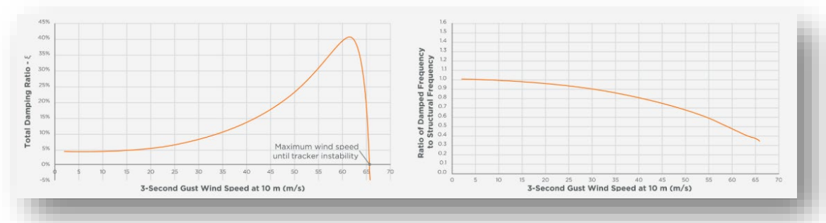
Figura 5 a sinistra FAM: rapporto di smorzamento/velocità del vento - a destra: rapporto di frequenza/velocità del vento
