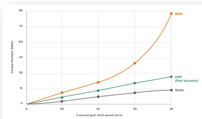
Figura 7 confronto tra carichi di vento statici e dinamici
