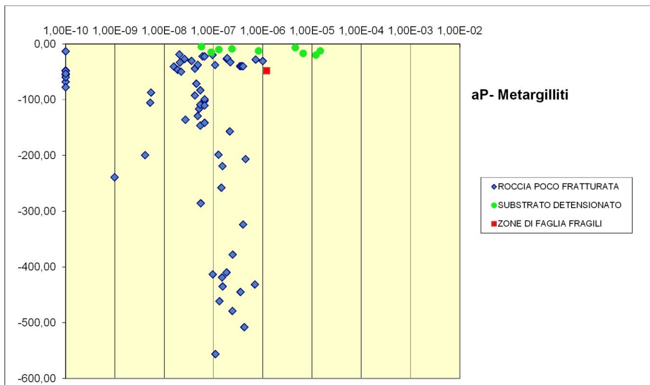
Figura 6 – Distribuzione dei valori di permeabilità ottenuti da prove in foro per gli argiloscisti dell'unità aP.
