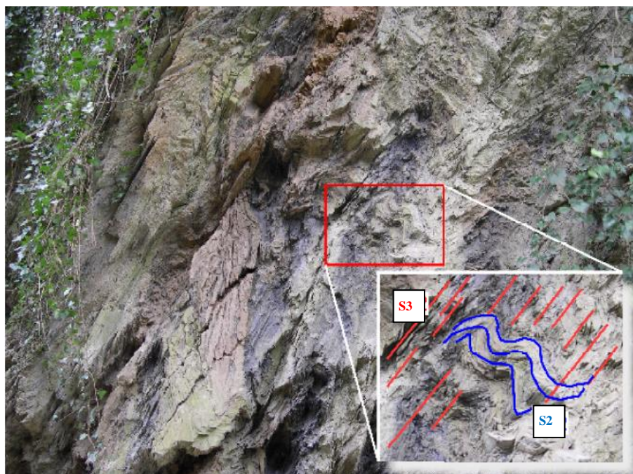
Figura 5 – Rapporti di sovrapposizione tra la scistosità composta principale (S1+S2) e clivaggi di piano assiale legati a pieghe aperte di fase D3 negli argilloscisti.
