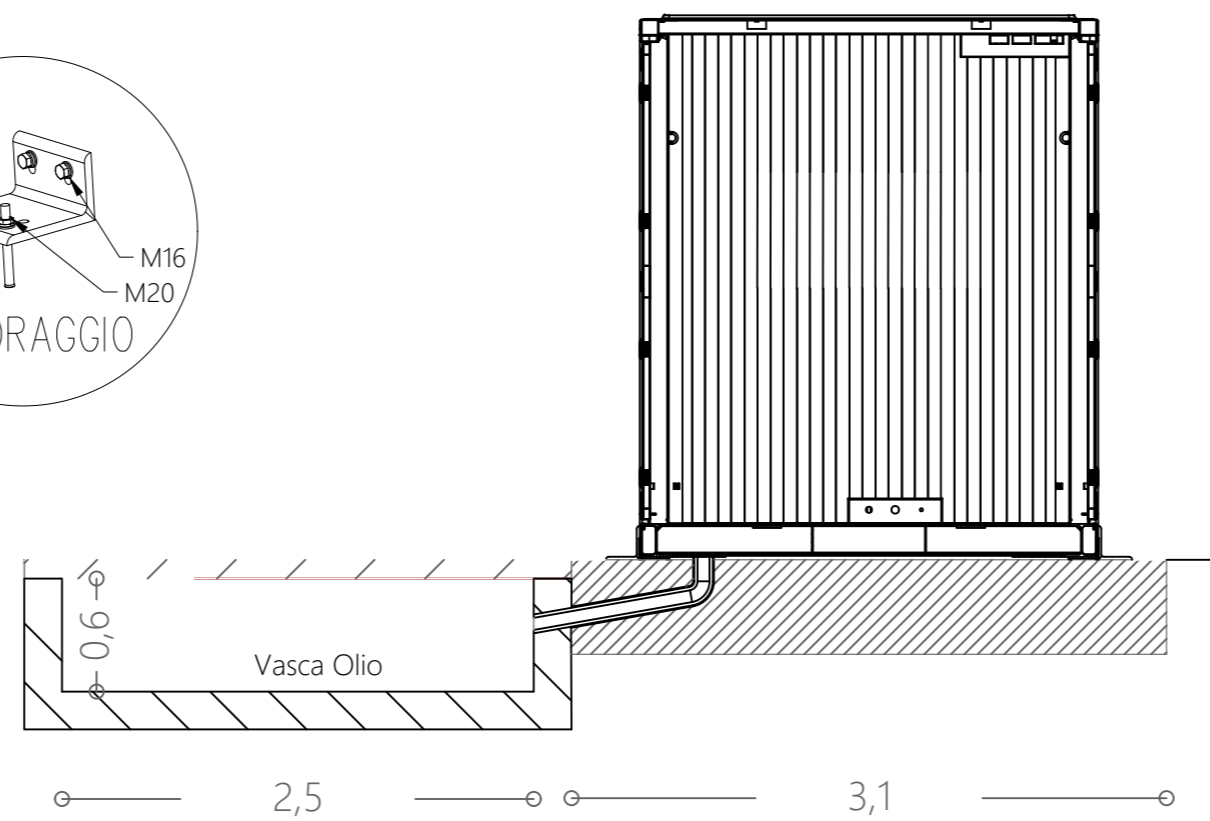
Sezione A-A
