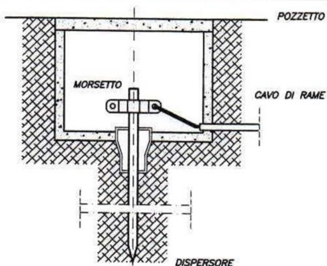
Figura 3-1 dispersore di terra con pozzetto ispezionabile
