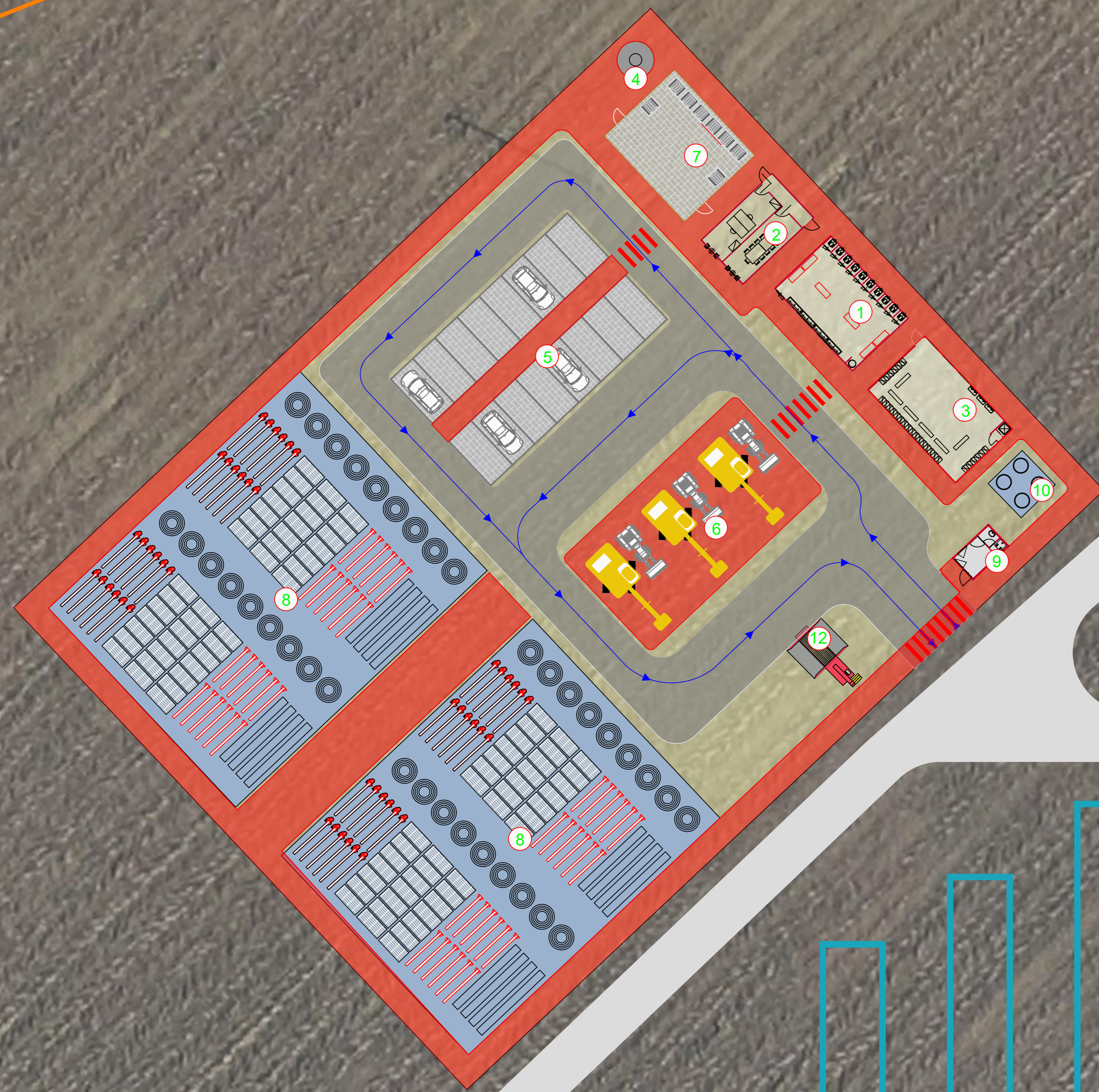
AREA DI CANTIERE 1 SCALA 1:250
