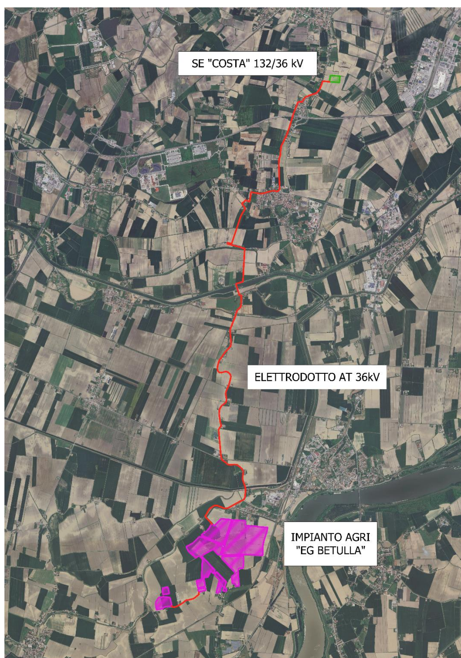
Figura 1 Ortofoto - impianto FV e connessione a futura SE.
