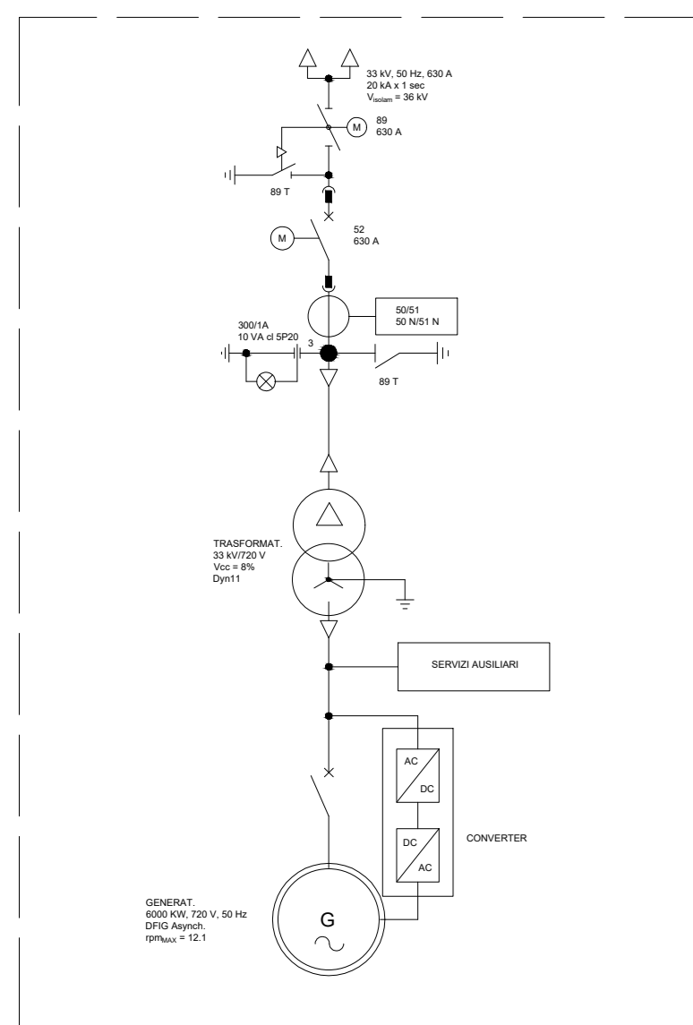
Dettaglio installazione a bordo torre di generazione eolica
