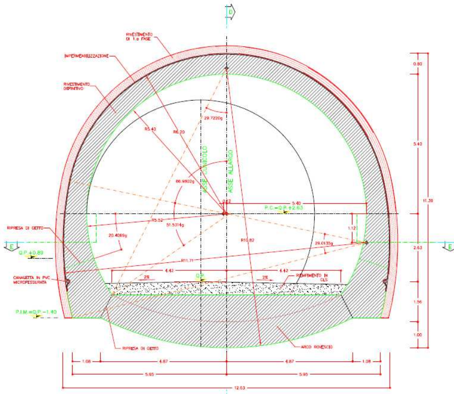
Sezione allargata
