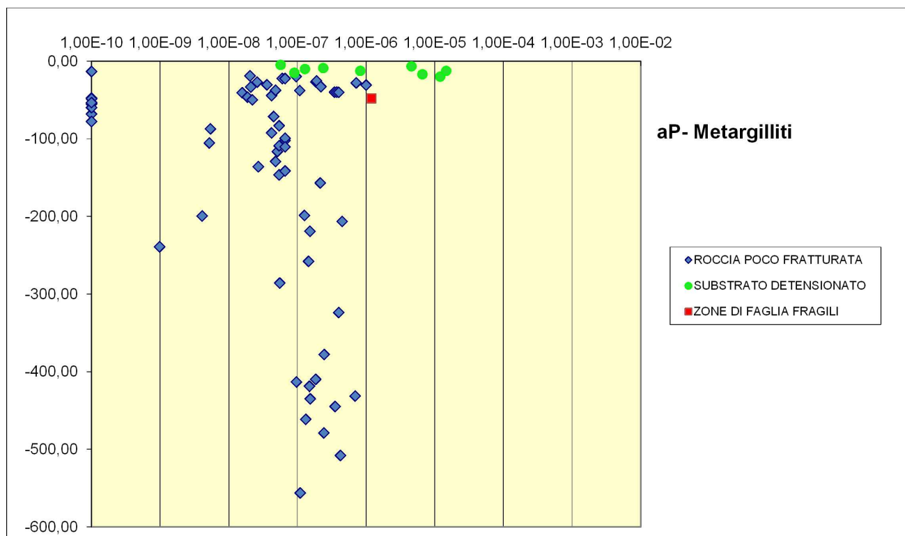
Figura 6 – Distribuzione dei valori di permeabilità ottenuti da prove in foro per gli argilloscisti dell'unità aP.
