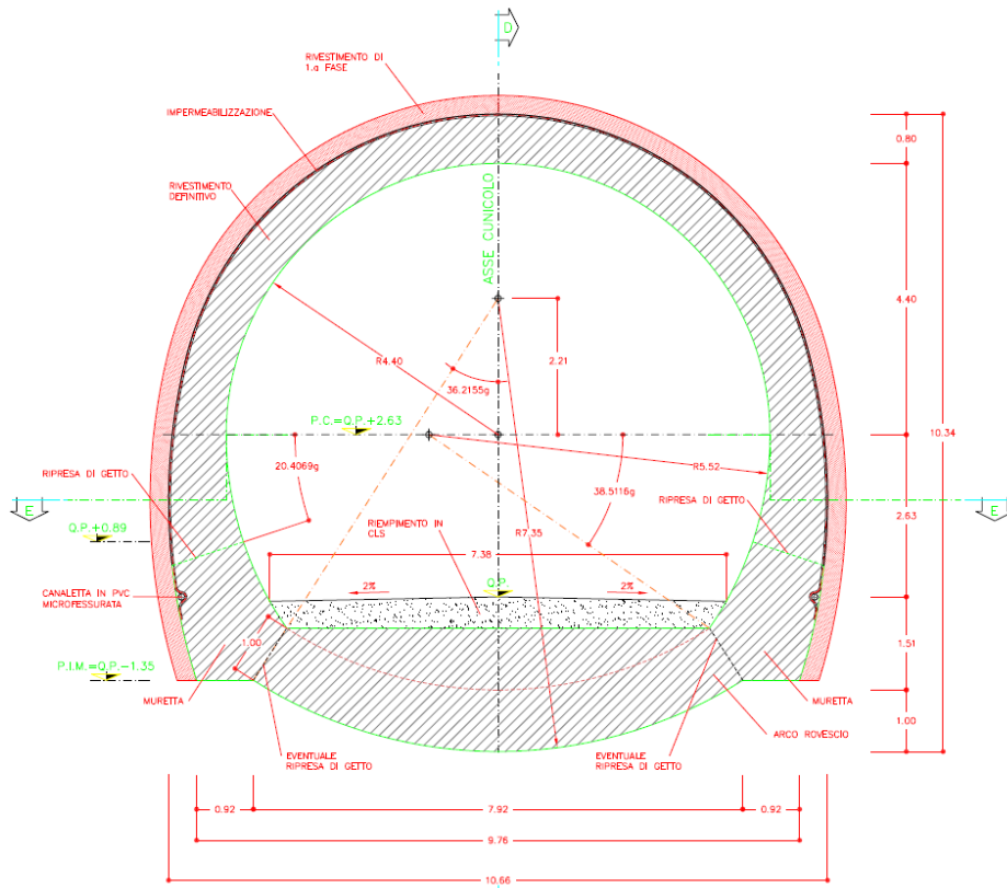
Sezione corrente
