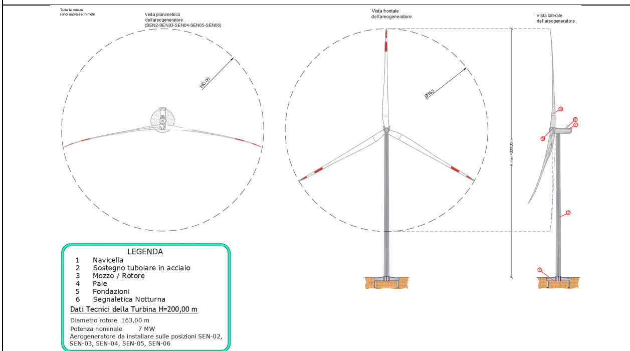
Figura 3-9 - Schema tipo aerogeneratore avente altezza al mozzo fino a 118,5 m e diametro rotore fino a 163 m per un'altezza complessiva di 200 m – cfr. elaborato SEN-PD-D25-00
