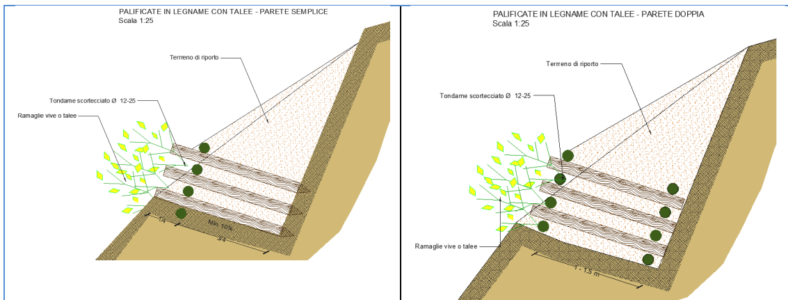
Figura 8.6 – Esempi di palificate in legname - Fonte HE
