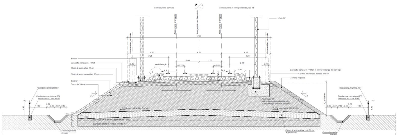
FIGURA 4 SEZIONE TIPO FERROVIARIA IN RILEVATO A DOPPIO BINARIO (PIATTAFORMA IN RETTO) CON HRIL ≤ 6,00 M
