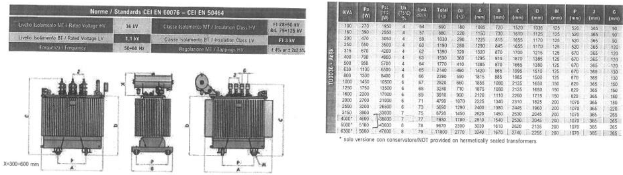
FIG. 11 – Datasheet Trasformatore
