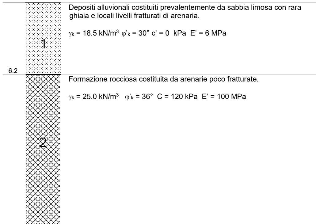
Figura 3.5/A: Schema stratigrafico e valori caratteristici dei parametri geotecnici
