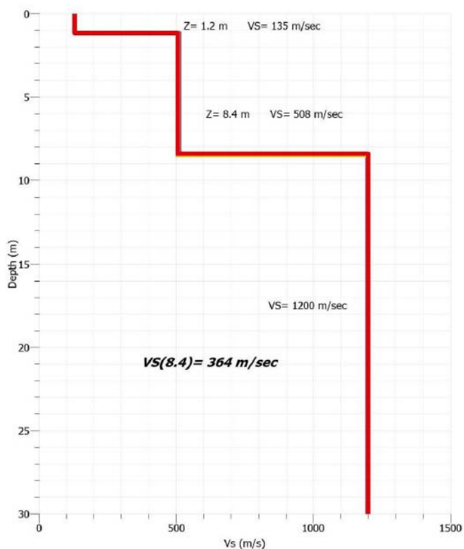
Figura 4.3/A: Profilo Vs-z ricavato dalla MASW VL-A-M16
