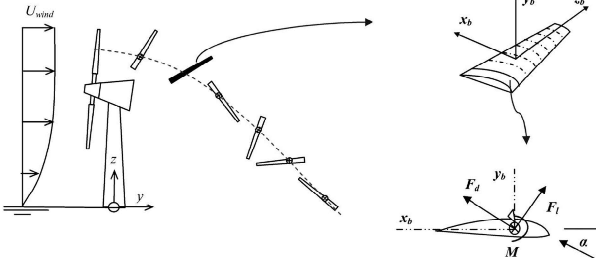
Immagine 1: schematizzazione del problema Sarlak, Sørensen: Analysis of throw distances of detached objects from horizontal-axis wind turbines. Wind Energy 2016;19; 153
