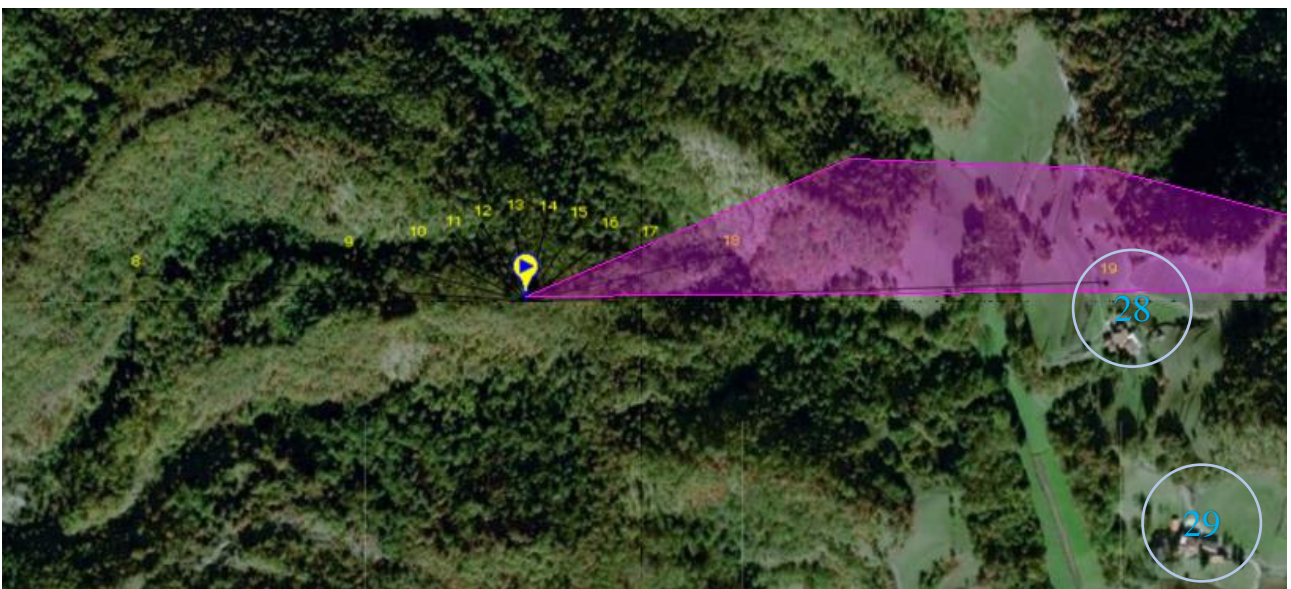
Figura 11: In magenta, azione ombreggiante generata da AG7 nel mese di settembre che coinvolge il recettore 28 tra le ore 18:00 e le 19:00.
