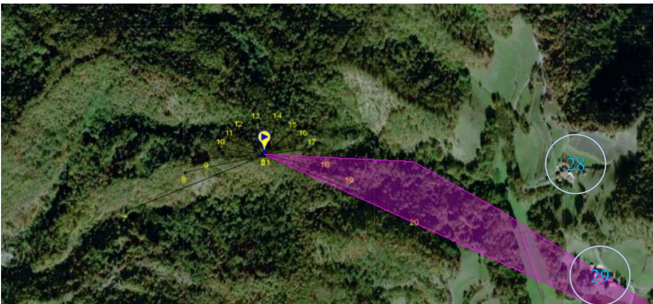
Figura 8: In magenta, azione ombreggiante generata da AG7 nel mese di giugno che coinvolge il recettore 29 tra le ore 18:00 e le 20:00.
