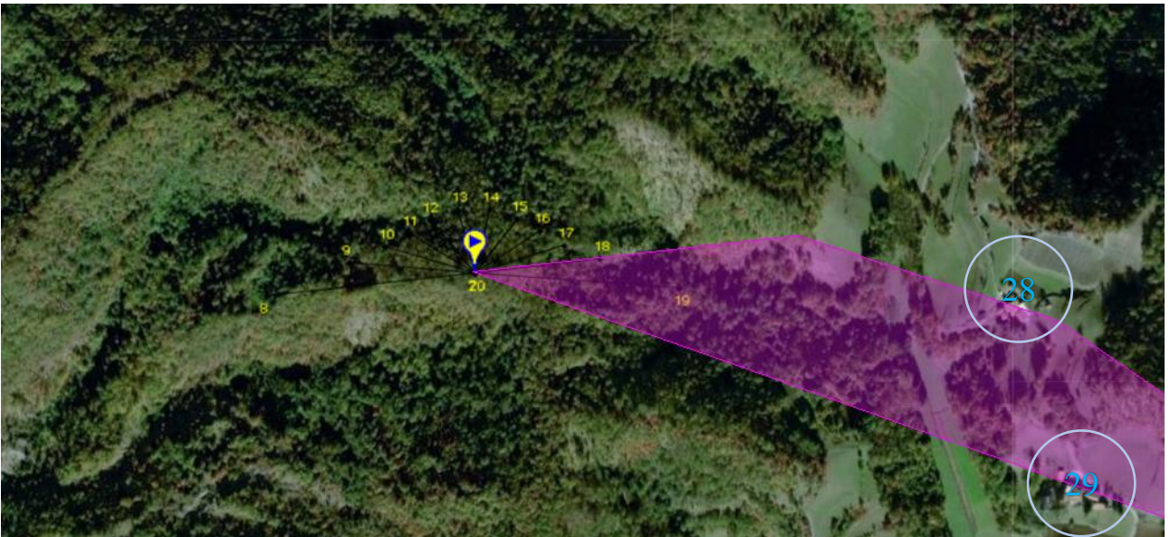
Figura 10: In magenta, azione ombreggiante generata da AG7 nel mese di agosto che coinvolge il recettore 28 e 29 tra le ore 19:00 e le 21:00.
