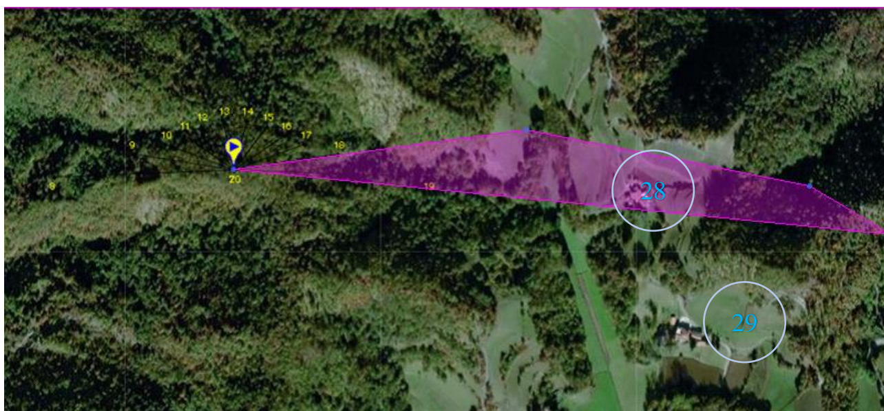
Figura 6: In magenta, azione ombreggiante generata da AG7 nel mese di aprile che coinvolge il recettore 28 tra le ore 18:00 e 20:00.
