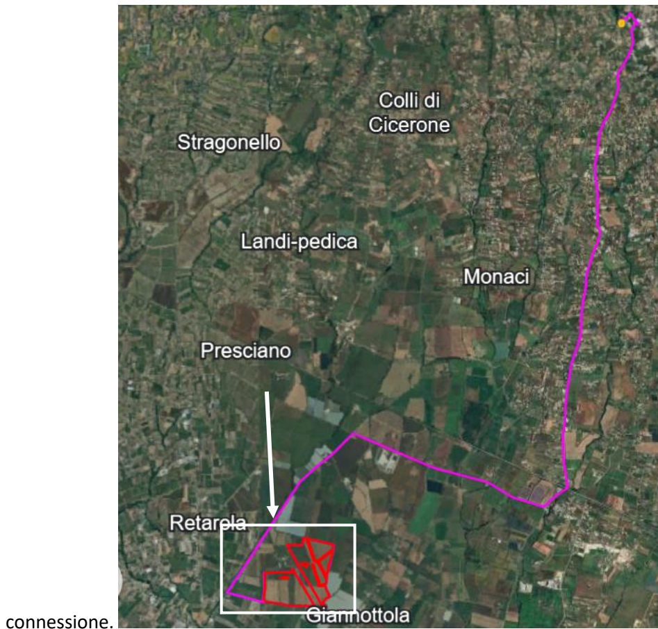
Fig.1 –Posizione impianto e cavidotto
