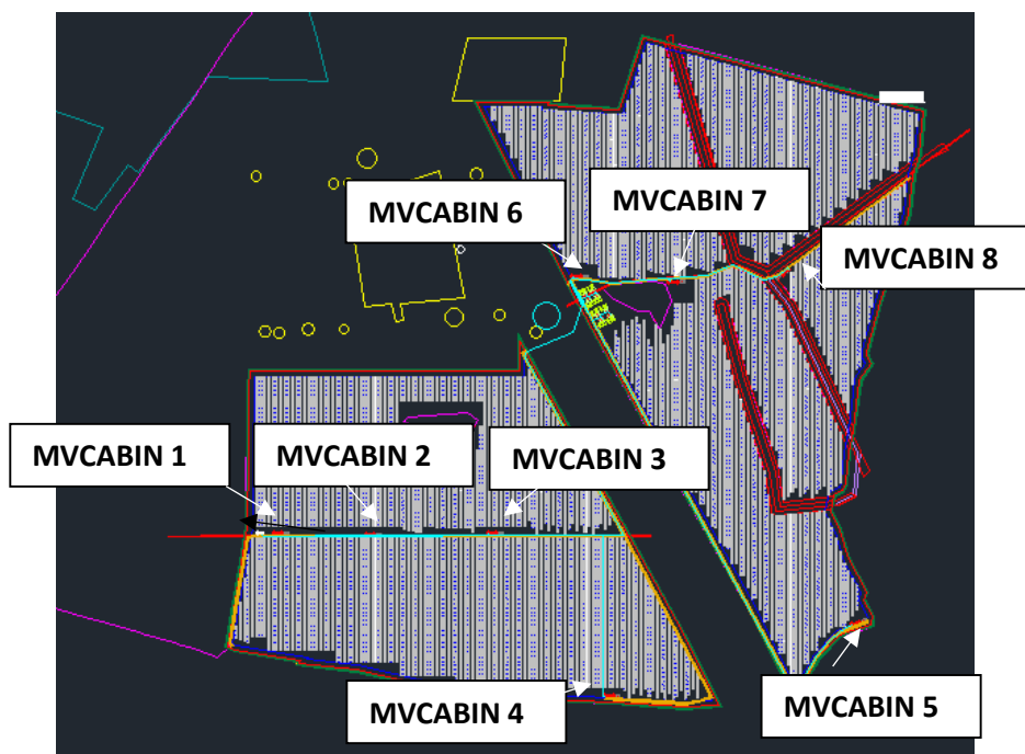
Fig.6– Impianto fotovoltaico posizione delle cabine
