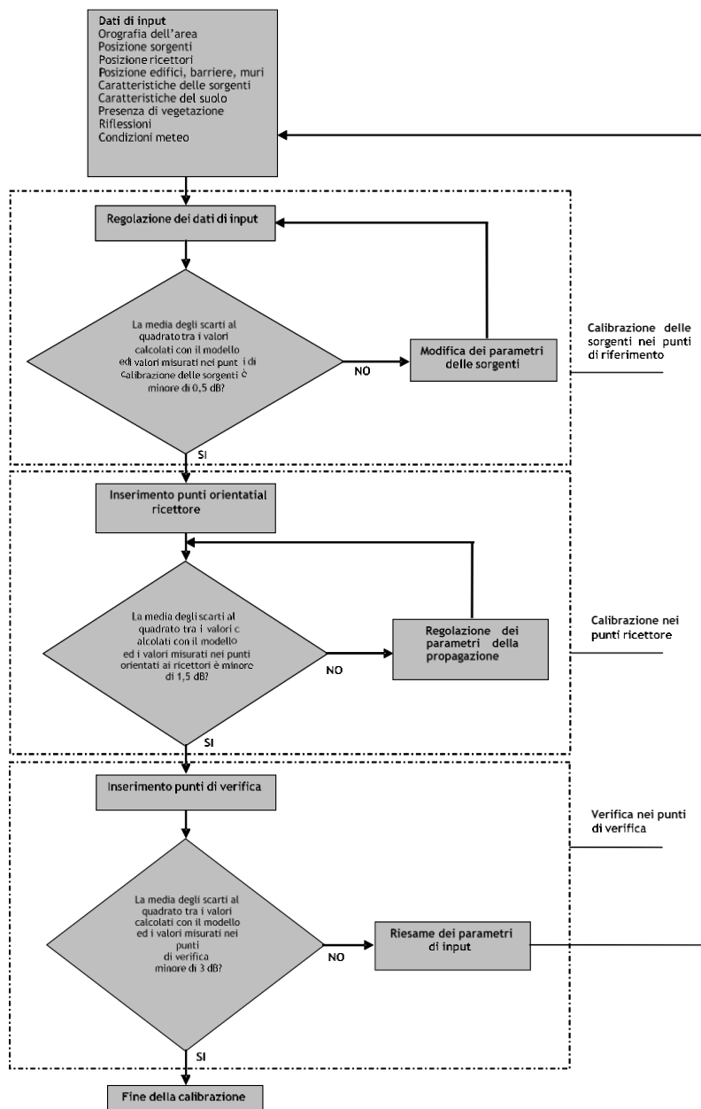
Fig. 11 – Schema a blocchi esemplificativo della procedura di calibrazione.
