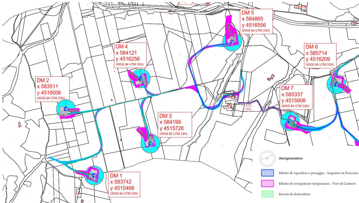
Figura 5 – Rappresentazione grafica generale aree di occupazione e servitù (1/2)
