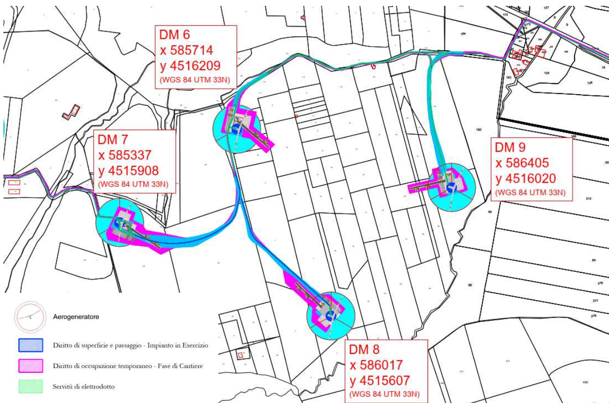
Figura 6 – Rappresentazione grafica generale aree di occupazione e servitù (2/2)
