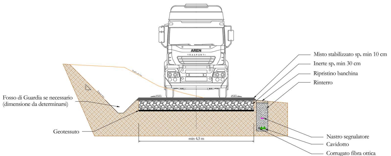
Figura 8 – Sezione tipo strade
