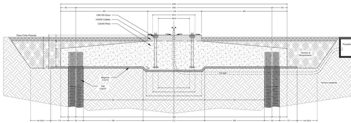
Figura 4 – Dettaglio sezione fondazione
