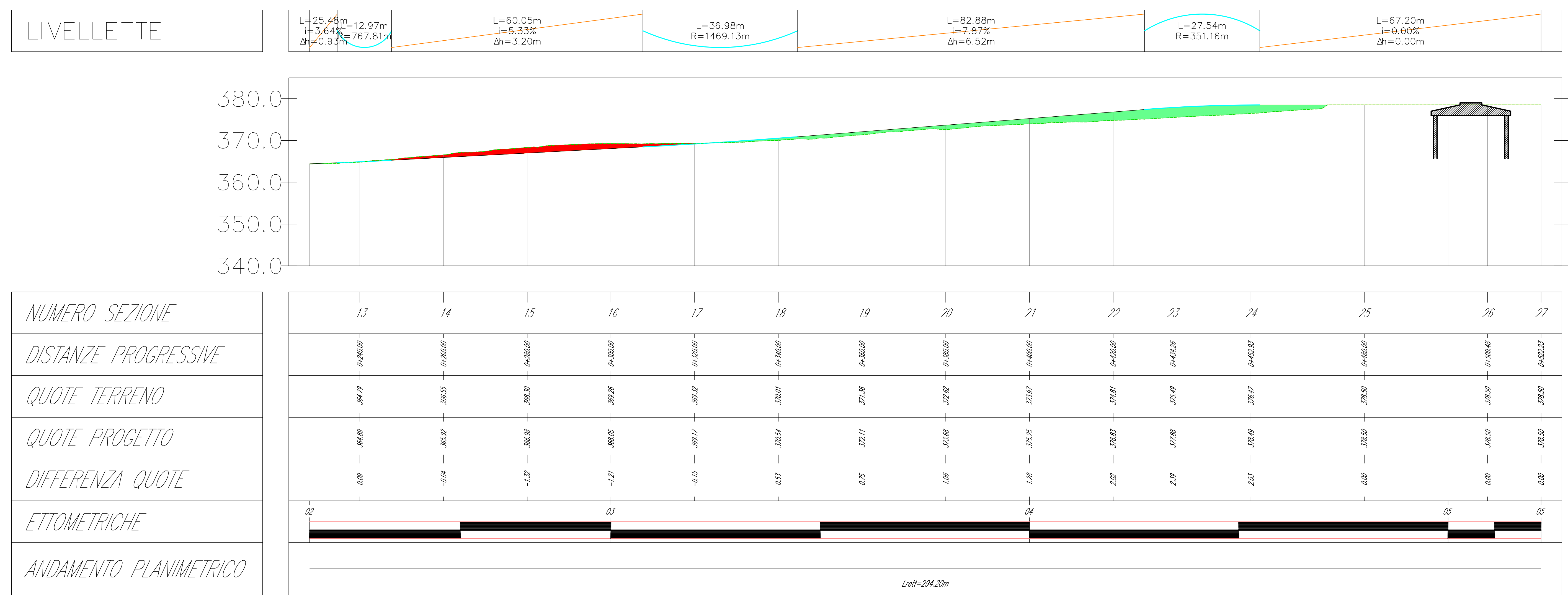
Profilo: Profilo Tracciato DM08 2 di 2 Q.Rif. : 340.00
