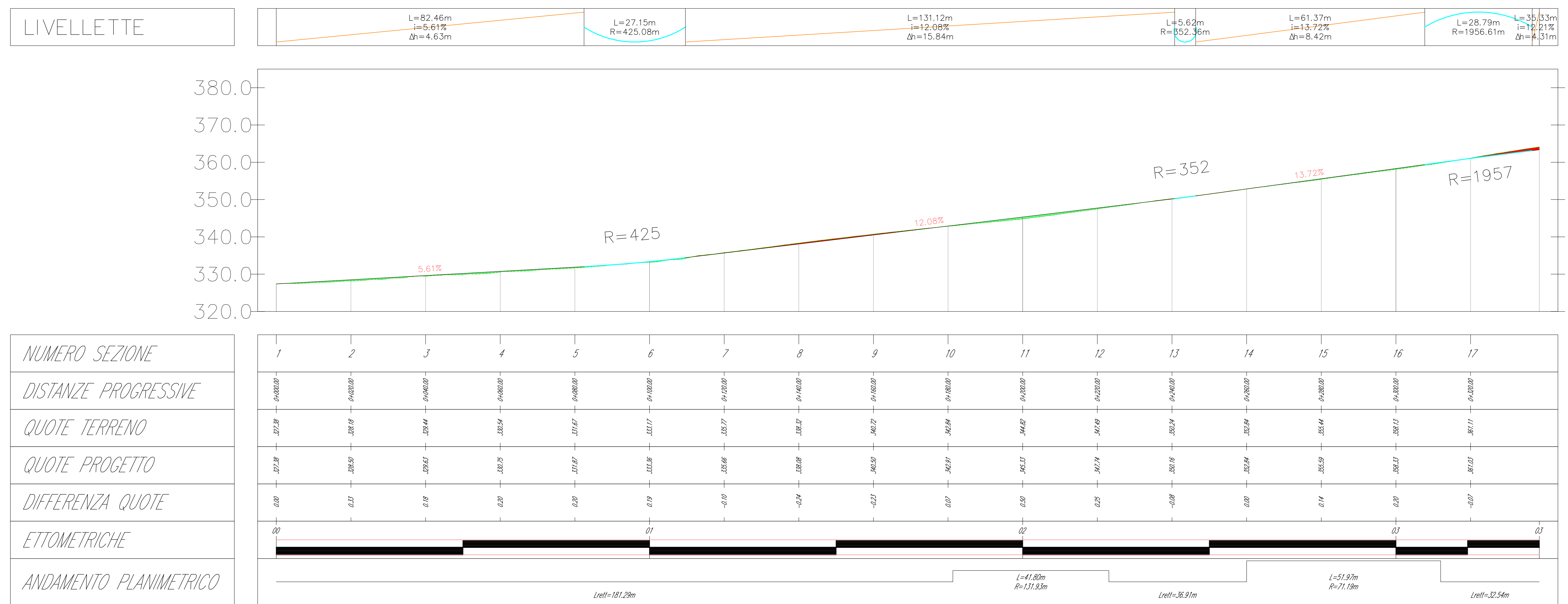
Profilo: Profilo Tracciato DM07 1 di 2 Q.Rif. : 320.00
