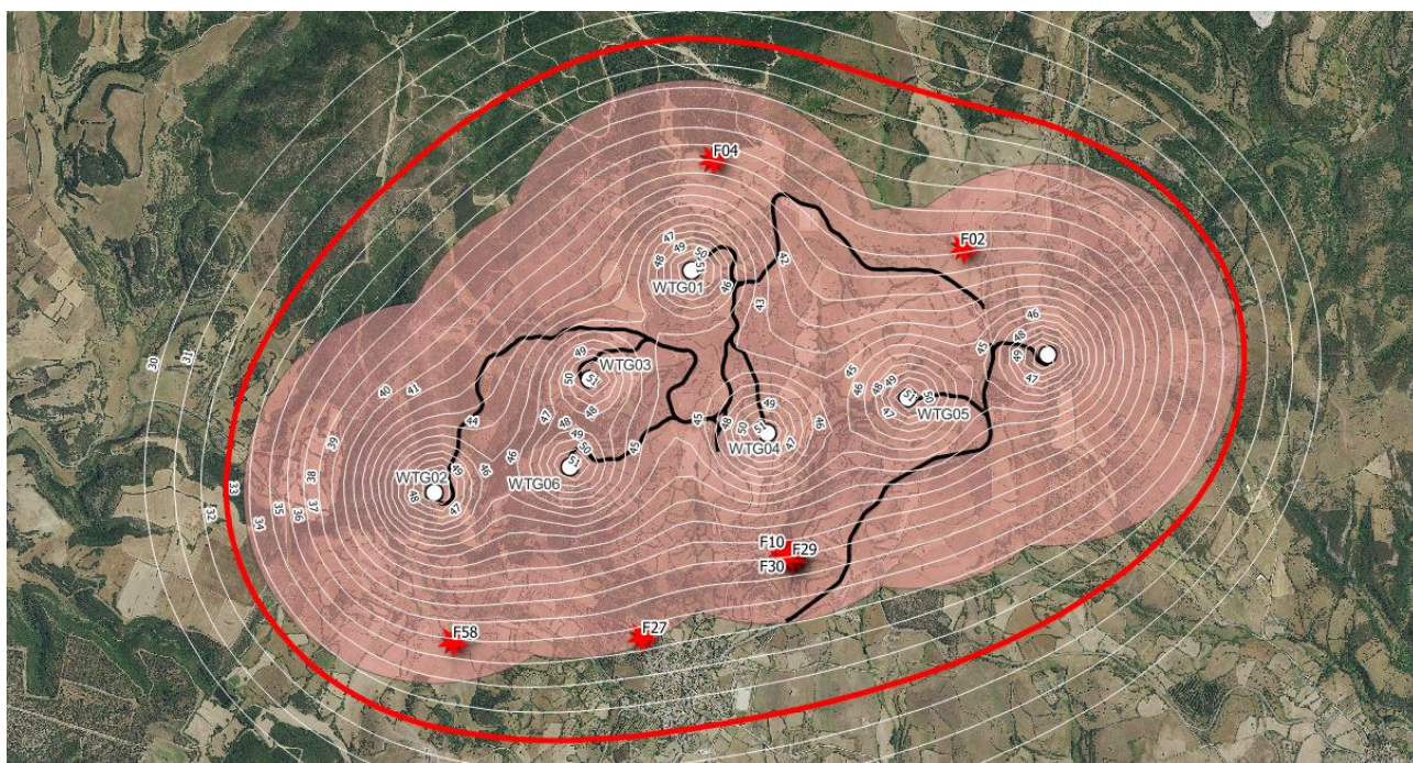
Figura 2.5 – Campo sonoro generato dall'impianto. In rosso l'isofonica dei 33 dB(A), attestata ad una distanza indicativa di 1.000 m dalle postazioni eoliche in progetto
